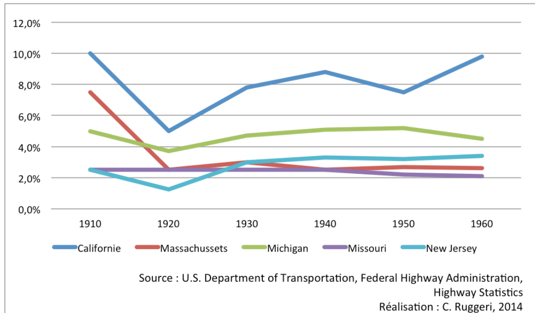
Graphique IV.7.1 – Part des immatriculations de cinq États entre 1910 et 1960 233
