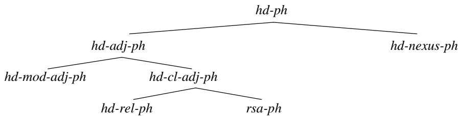
Figure 5 – Hiérarchie (partielle) des super-types du type rsa-ph
