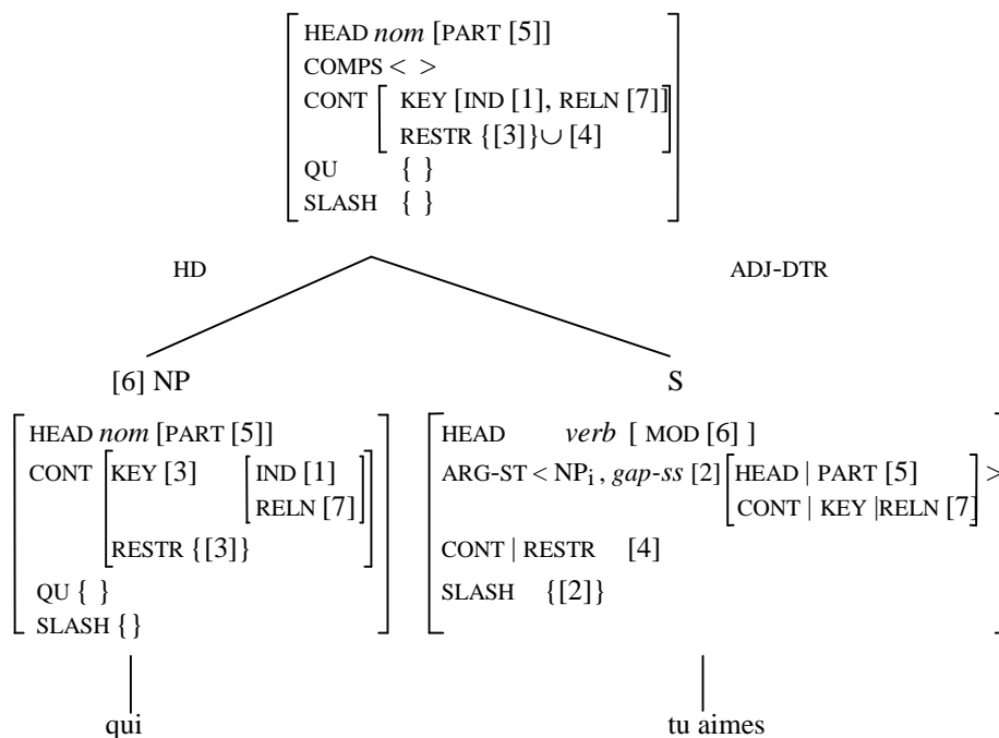
Figure 7 – Description partielle pour la RSA ( j'aime ) qui tu aimes
