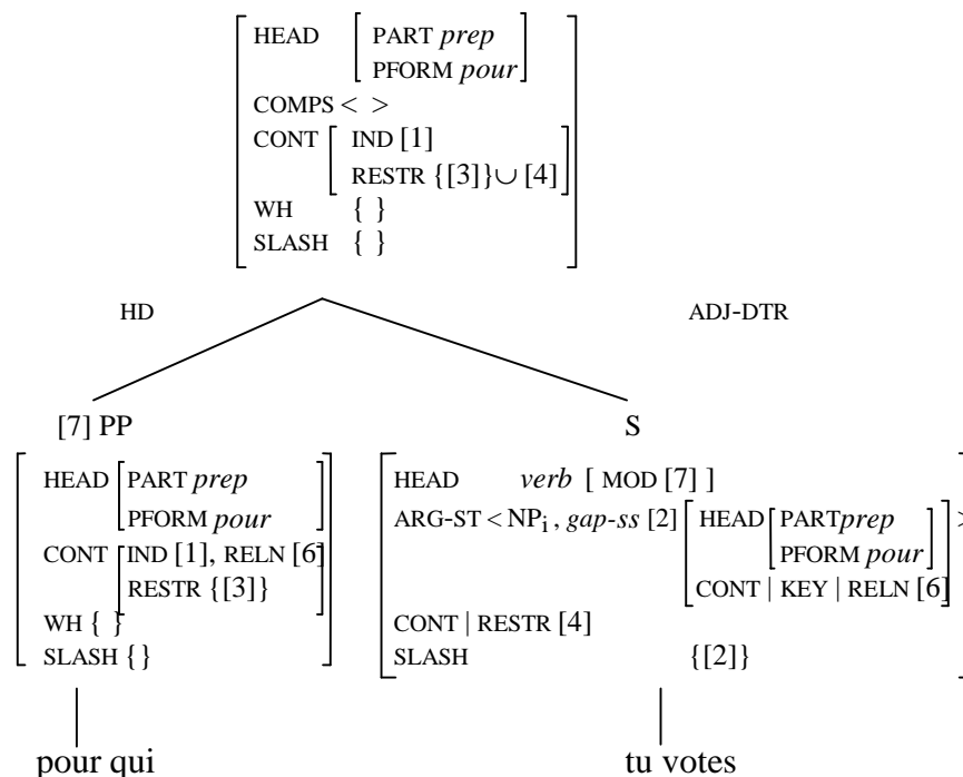
Figure 8 – Description partielle pour ( Paul votera ) pour qui tu votes
