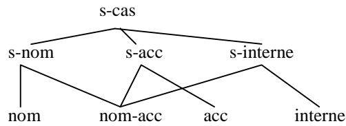
Figure 10 – Hiérarchie des cas directs pour le français
