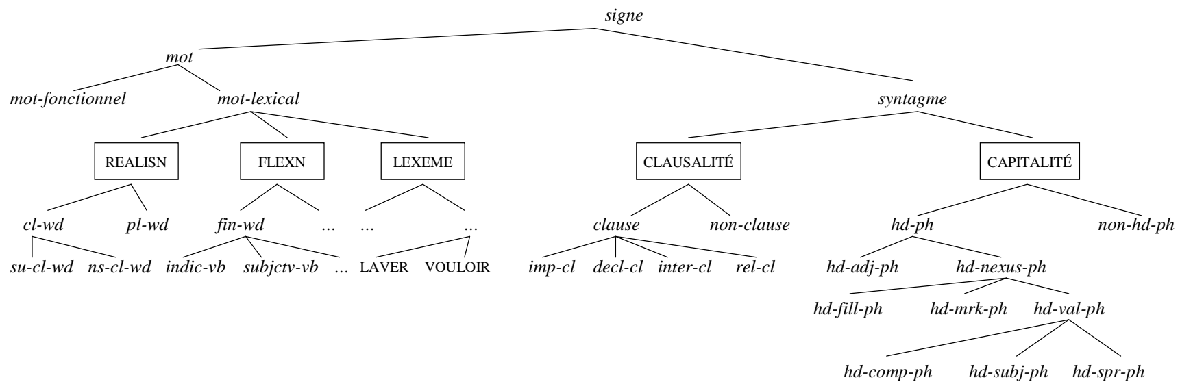
Figure 2 – Hiérarchie typée des objets de type signe
