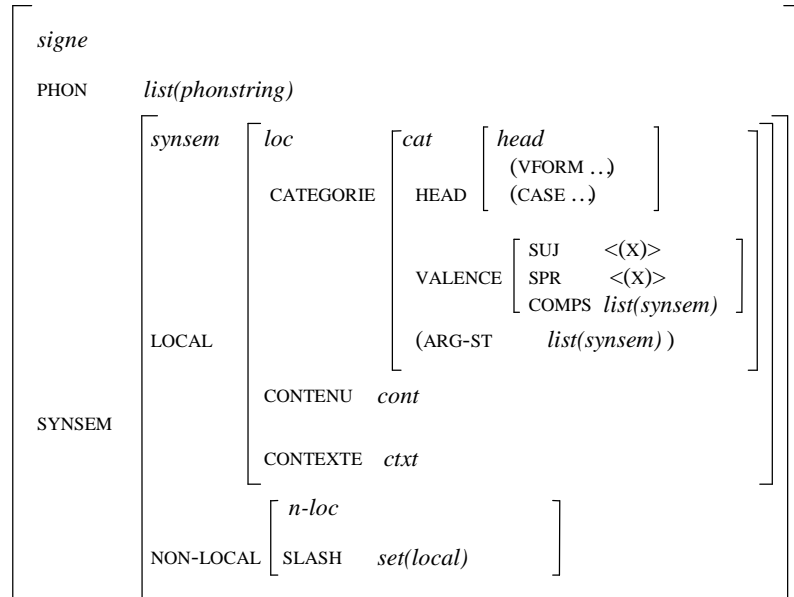
Figure 1 – Structure de traits pour un objet de type signe
