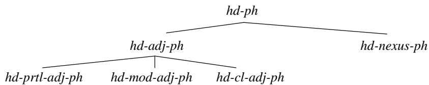
Figure 1 – Hiérarchie (partielle) des sous-types de hd-adj-ph
