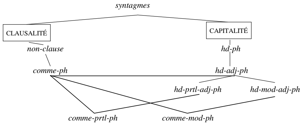
Figure 2 – Hiérarchie des sous-types de comme-ph
