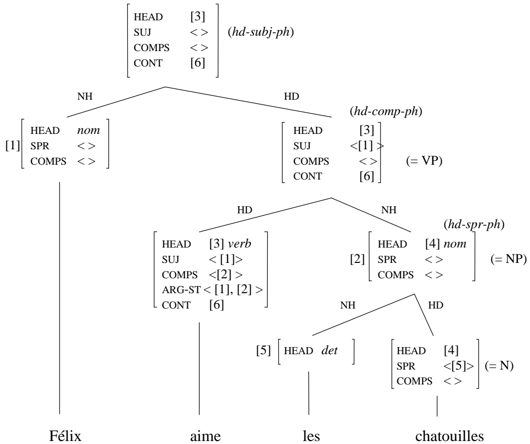
Figure 3 – Description partielle d'une phrase simple
