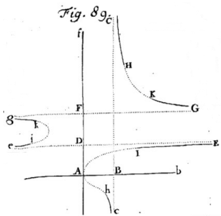
FIGURE 6.14 – Branches infinies, cas II : exemple de la courbe d'équation xyy - ayy - 3axy + 2a^2x = 0 (p. 262 et Planche XII figure 89, p. 274).
