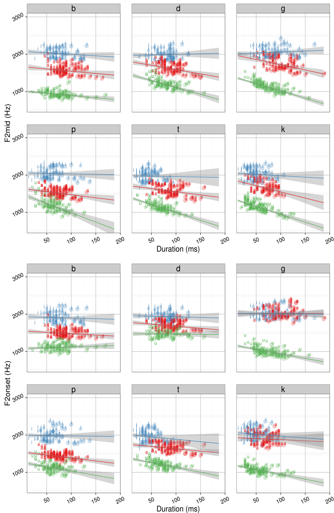
FIGURE 6.5 – Représentation de la variation des F2_{mid} (en haut) et des F2_{onset} (en bas) en fonction du temps dans chaque contexte consonantique initial pour les cinq locuteurs. Les cercles transparents de tailles différentes entourant les voyelles désignent qu’elles sont réalisées dans un débit lent (grands cercles) et moyen (petits cercles). L’absence de cercles indiquent que les voyelles sont prononcées dans un débit rapide.
