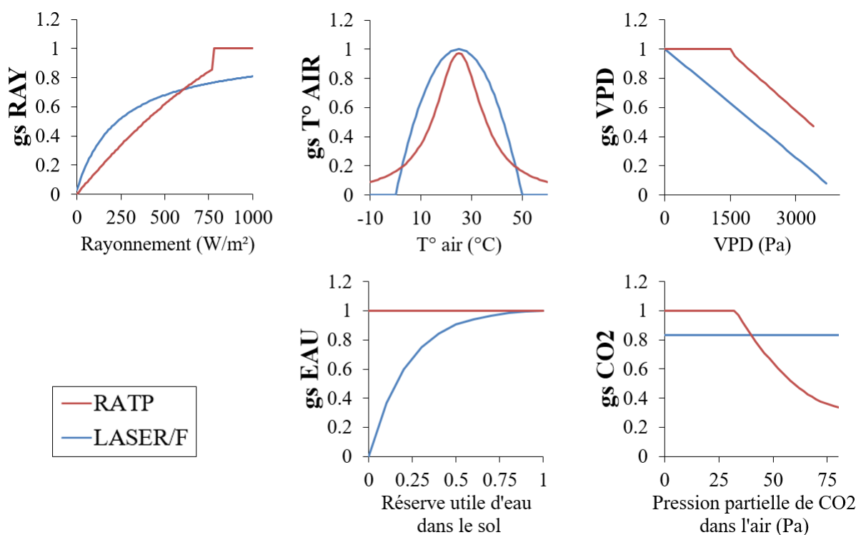
Figure 4.1 – Conductance stomatique (gs) de chaque modèle, RATP (en rouge) et LASER/F (en bleu) en fonction de facteurs météorologiques : rayonnement (RAY - \text{W}/\text{m}^2 ), température de l'air ( T^\circ\text{AIR} - ^\circ\text{C} ), déficit de pression de vapeur d'eau (VPD - Pa), réserve utile d'eau dans le sol (EAU) et pression partielle de \text{CO}_2 dans l'air ( \text{CO}_2 - Pa).
