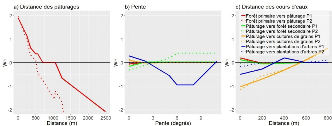
Figure 115. Valeurs de W^+ en fonction des variables distance aux pâturages, pente et distance aux rivières principales pour les principales transitions de l'occupation du sol dans les phases P1 (t0, 2004 ; t1, 2007) et P2 (t0, 2010 ; t1, 2013).
