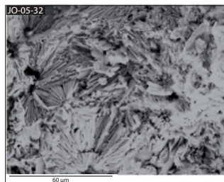
h-Précipitation radiale de cristaux fibreux autour de petites sphérules (MEB).
