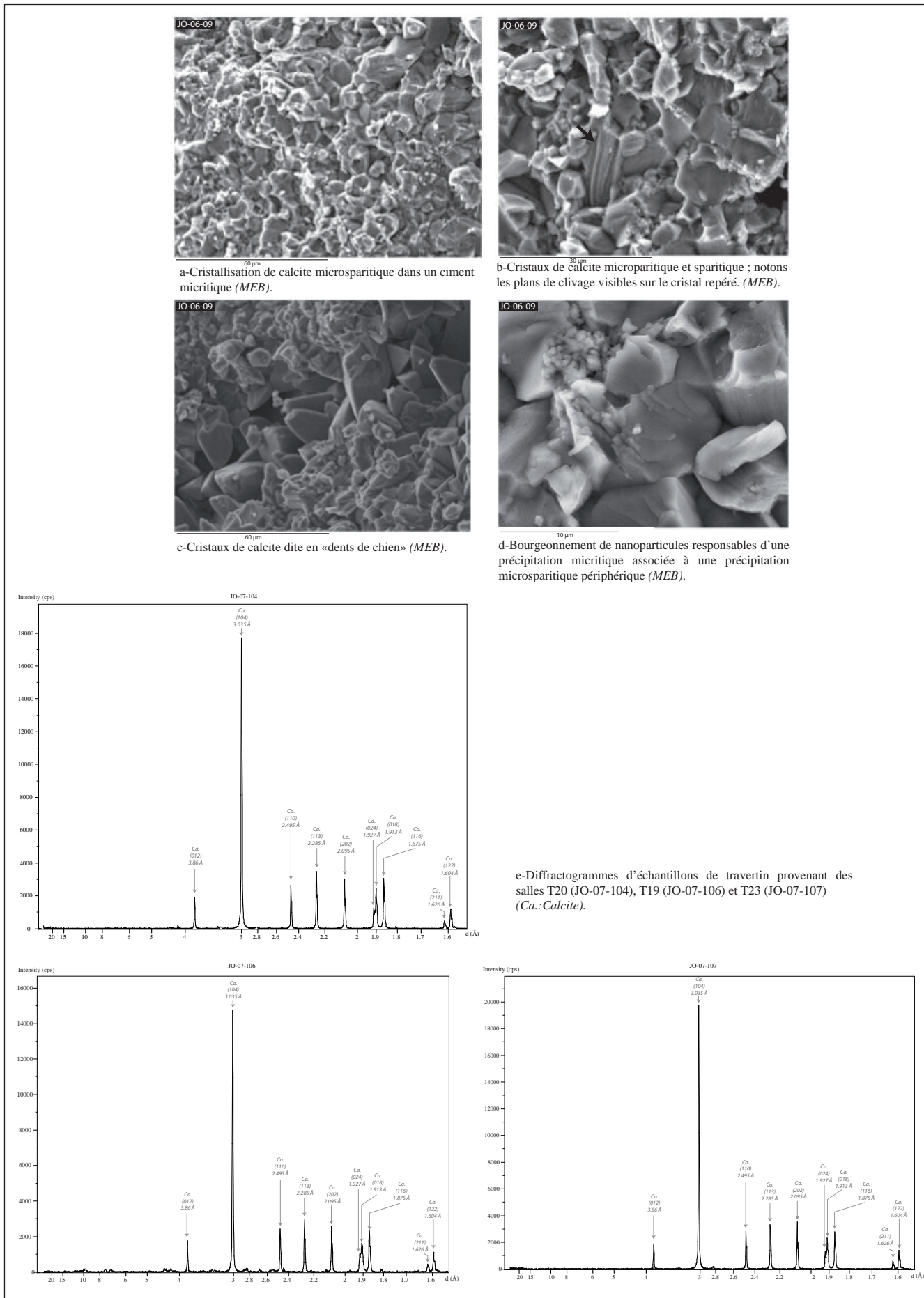
Figure B.72. Plaque pétrographique (images MEB et DRX, suite de la Fig. B.71) du faciès C défini dans les thermes antiques de Jebel Oust ; voir les commentaires dans le texte.
