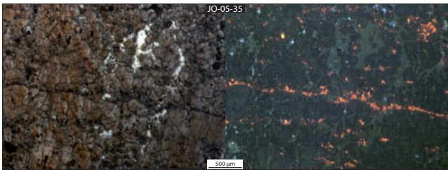
g-Botryoides aragonitiques (non-luminescent) et lamine calcitique (luminescent) (gauche : LN ; droite : IC).
