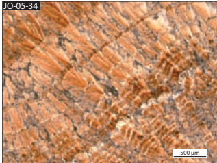
e-Alternance de lamines sparitiques à grands cristaux rayonnants et de lamines micritiques (LN).
