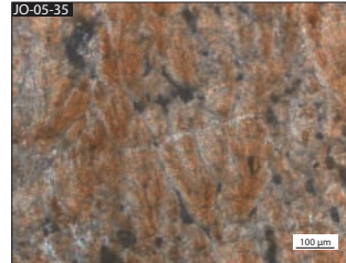
f-Cristaux sparitiques buissonnants ( shrub crystals ) (LP).
