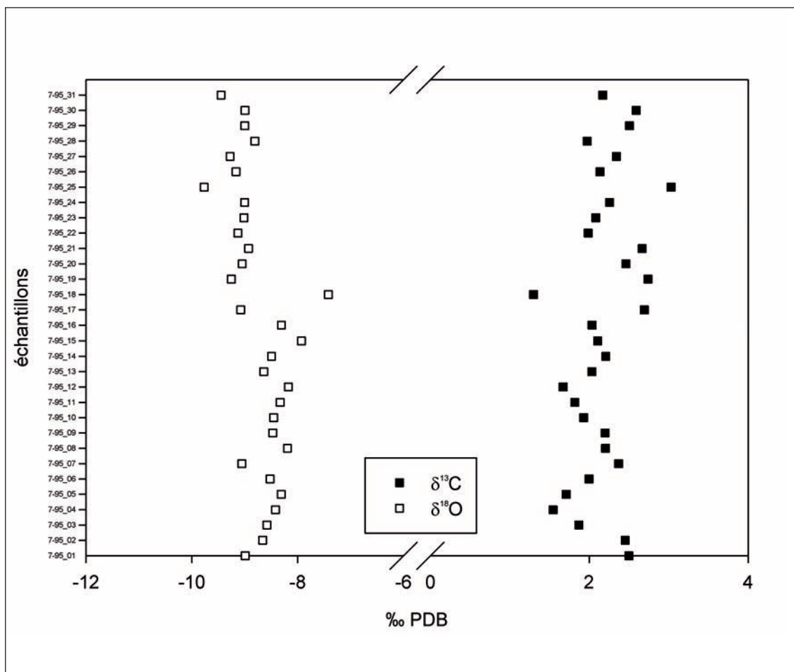
Figure B.45. Évolution des valeurs de \delta^{18}\text{O} et de \delta^{13}\text{C} le long de l'échantillon laminé JO-07-95 de l'aqueduc thermal de Jebel Oust.
