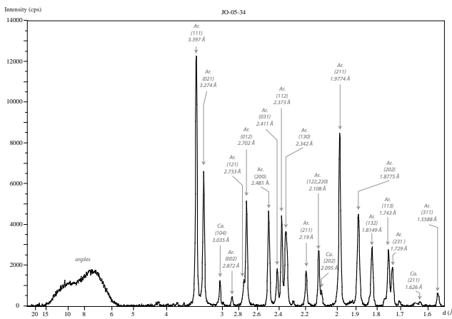
k-Diffractogramme d'échantillons de travertin provenant de la salle T1 (JO-05-34) et T7 (JO-07-114) ; (Ar.:Aragonite ; Ca.:Calcite).
