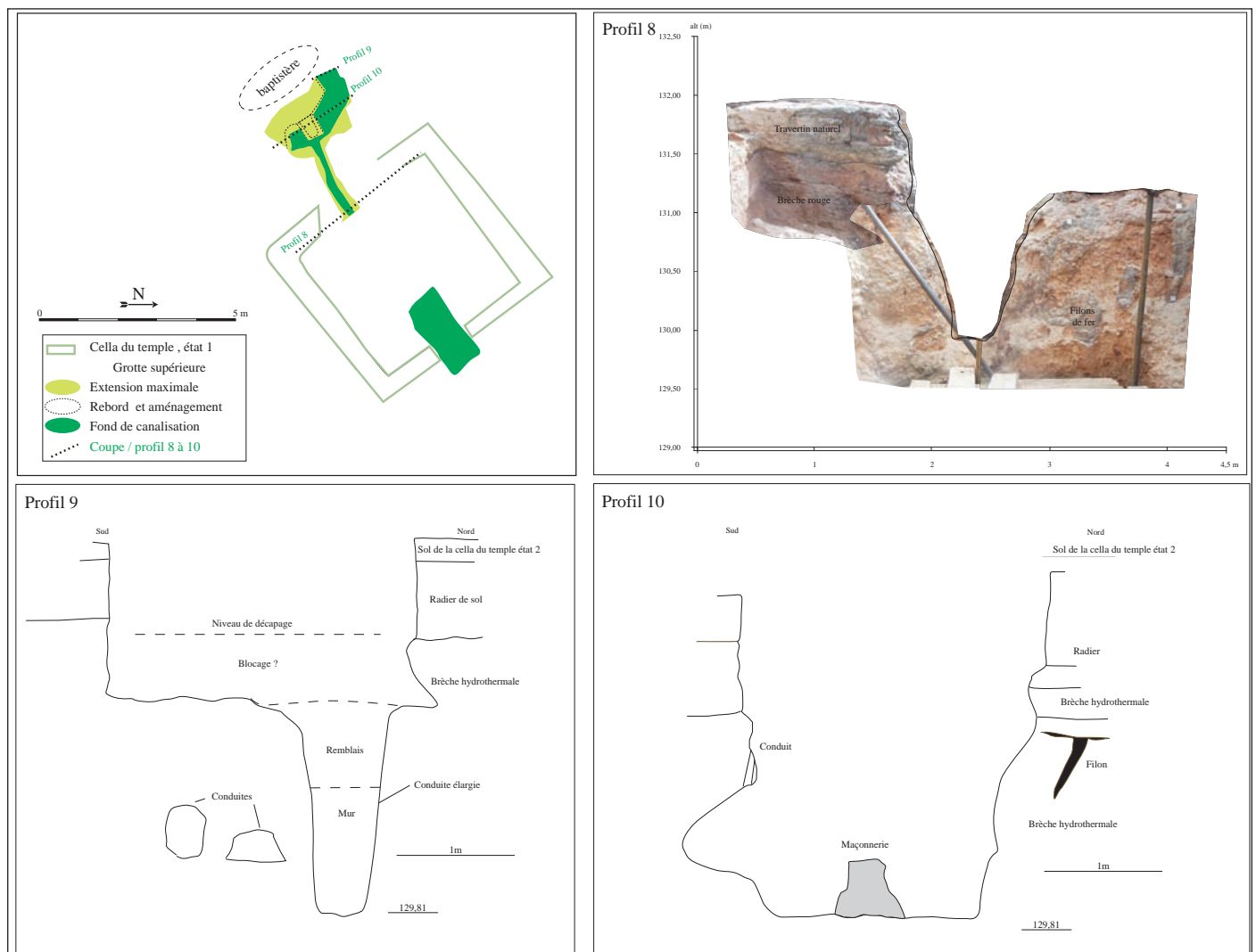
Figure B.50. Plan du captage supérieur de la source chaude antique (premier captage) et profils topographiques associés.
