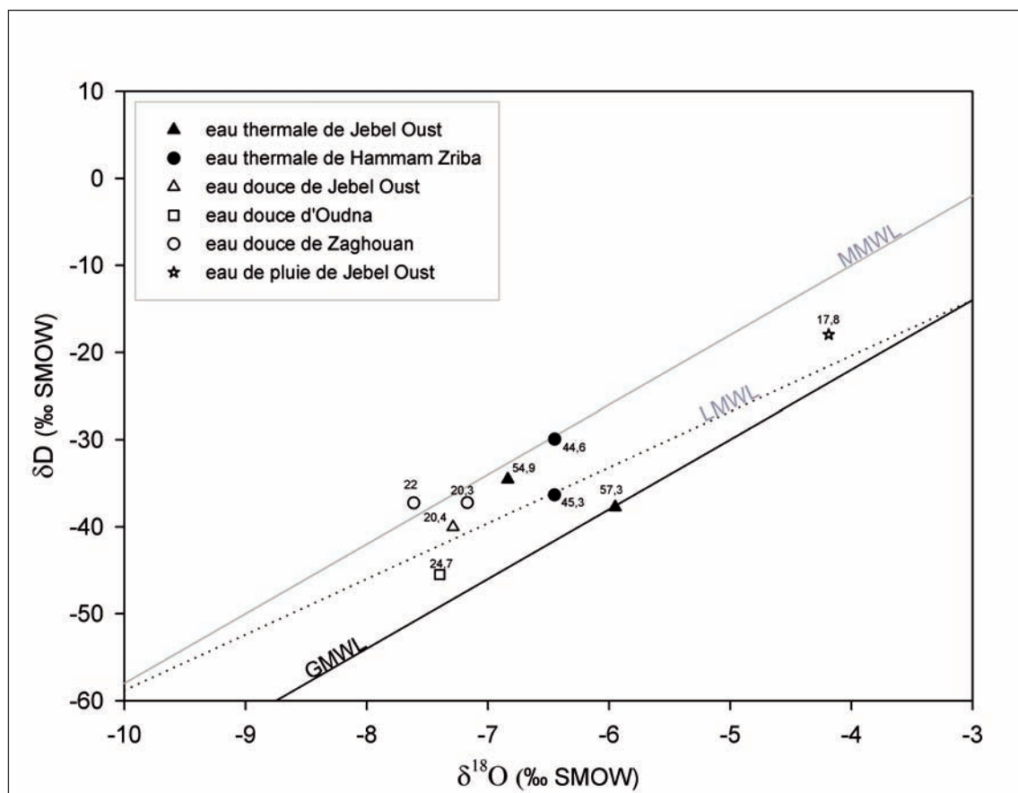
Figure B.36. Diagramme \delta^{18}\text{O}/\delta\text{D} des eaux de la région de Jebel Oust (et températures associées en °C) ; GMWL = Global Mean Water Line (Craig, 1961), LMWL = Local Mean Water Line (Celle-Jeanton et al., 2001), MMWL = Mediterranean Mean Water Line (Sadki, 1998).
