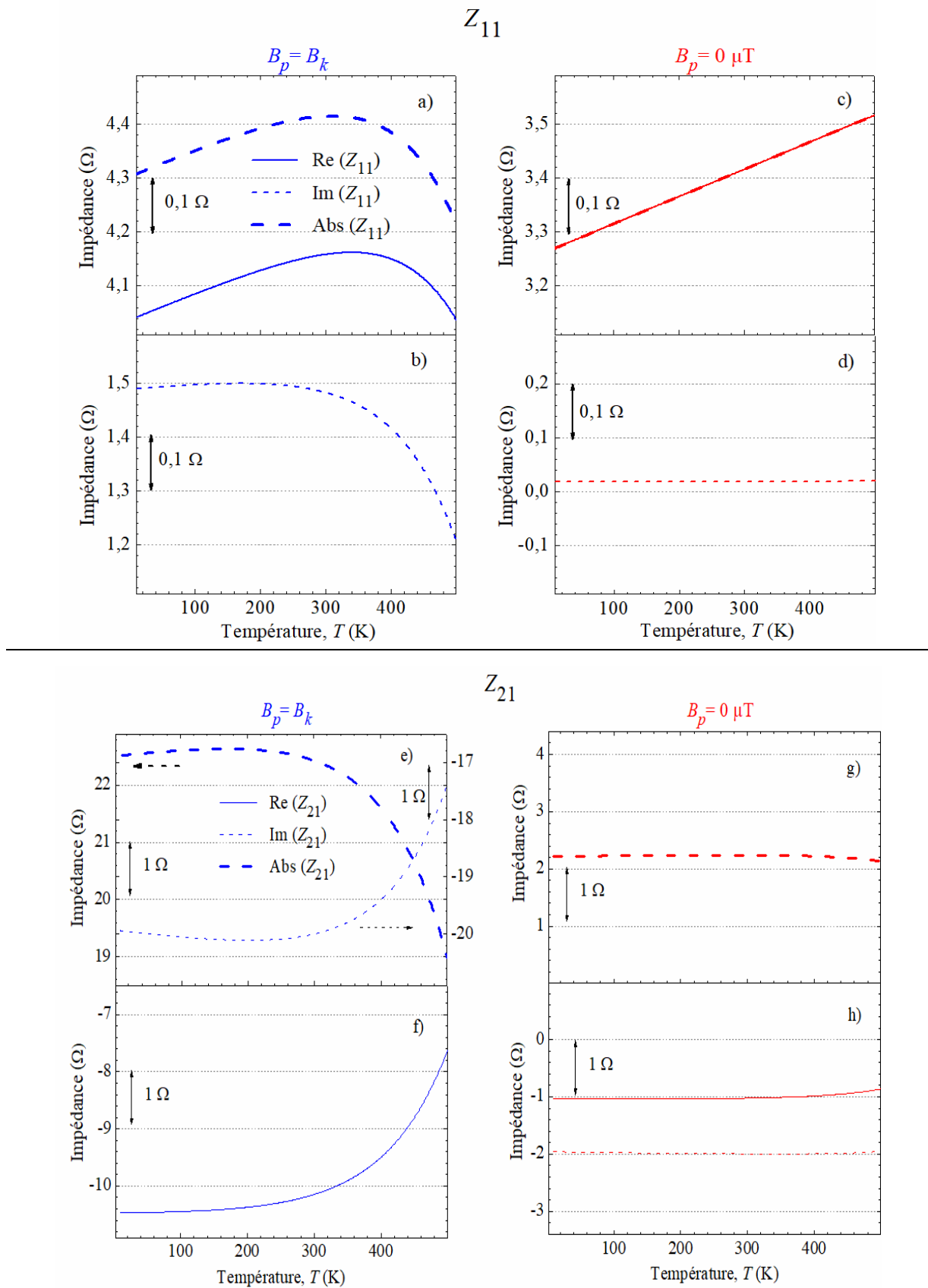
Figure 3.8 : Variations des parties réelles (courbes pleines), imaginaires (courbes pointillées) et absolues (courbes pointillées en gras) de l'impédance diagonale (graphs a), b), c) et d) et off-diagonal (e), f), g) et h)) en fonction de la température. Les courbes bleues correspondent à B_p = B_k et les courbes rouges correspondent à B_p = 0 \mu\text{T} .
