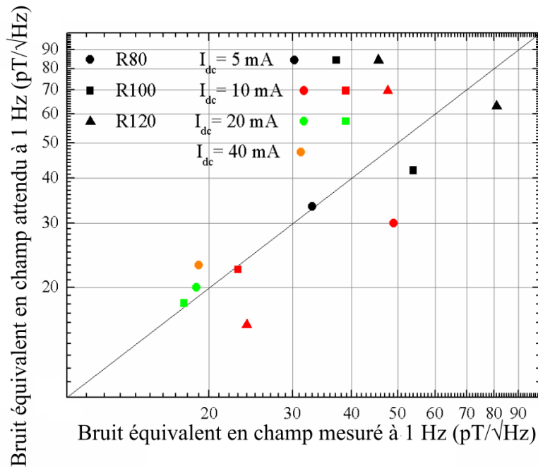
Figure 2.7 : Bruit équivalent en champ mesuré et calculé à partir de l'équation (2.3) pour les trois \mu fil MIG étudiés et pour différents courants statiques. La ligne noire représente une correspondance parfaite entre les valeurs calculées et mesurées de b_n .
