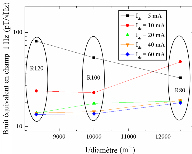
Figure 2.8: Présentation de l'évolution du niveau de bruit équivalent en champ, b_n , en fonction du diamètre des \mu fil MIG et du courant statique.
