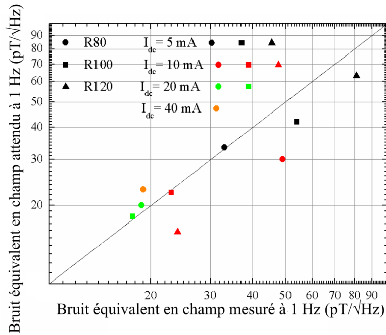
Figure 2.7 : Bruit équivalent en champ mesuré et calculé à partir de l'équation (2.3) pour les trois \mu fils MIG étudiés et pour différents courants statiques. La ligne noire représente une correspondance parfaite entre les valeurs calculées et mesurées de b_n .
