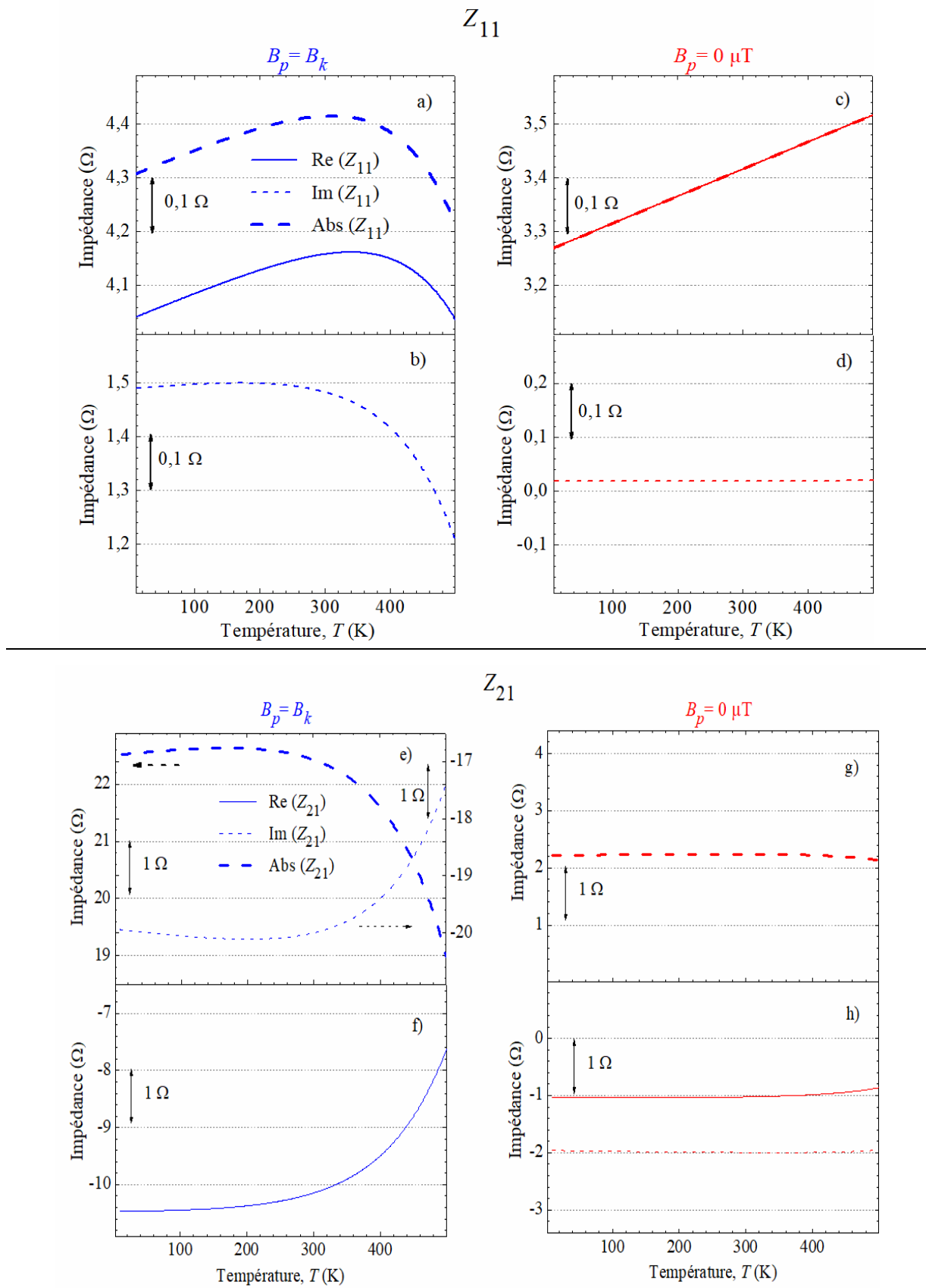
Figure 3.8 : Variations des parties réelles (courbes pleines), imaginaires (courbes pointillées) et absolues (courbes pointillées en gras) de l'impédance diagonale (graphs a), b), c) et d)) et off-diagonal (e), f), g) et h)) en fonction de la température. Les courbes bleues correspondent à B_p = B_k et les courbes rouges correspondent à B_p = 0 \mu\text{T} .
