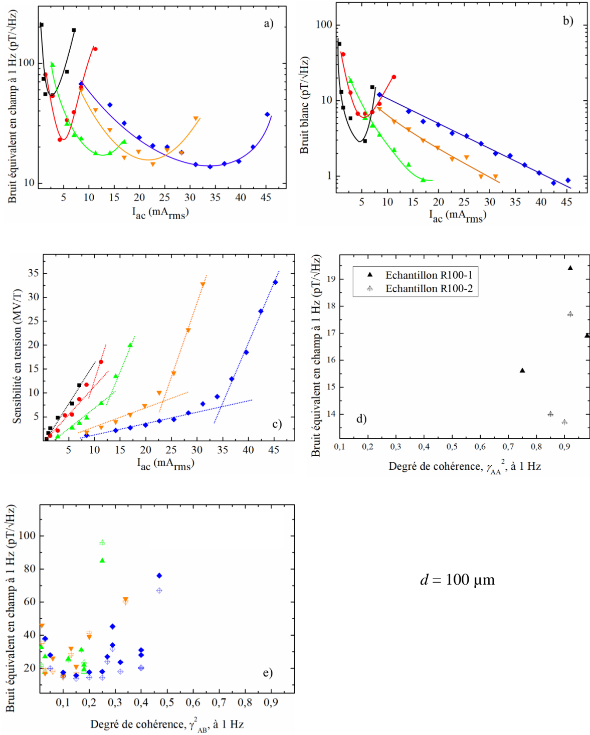
Figure 2.5 : Résultats expérimentaux montrant l'évolution du niveau de bruit équivalent en champ a) à 1 Hz et b) en zone de bruit blanc (en pT/ \sqrt{Hz} ), c) la fonction de transfert (en MV/T) et d) b_n à 1 Hz en fonction de la fonction de cohérence \gamma_{AA}^2 (en pT/ \sqrt{Hz} ) et e) \gamma_{AB}^2 pour deux échantillons (R100-1 et R100-2) de diamètre 100 \mu m . Les lignent servent uniquement de guides visuels.
