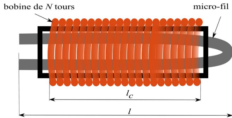
Figure 1.9 : Configuration d'un Fluxgate orthogonal en mode fondamental [44]
