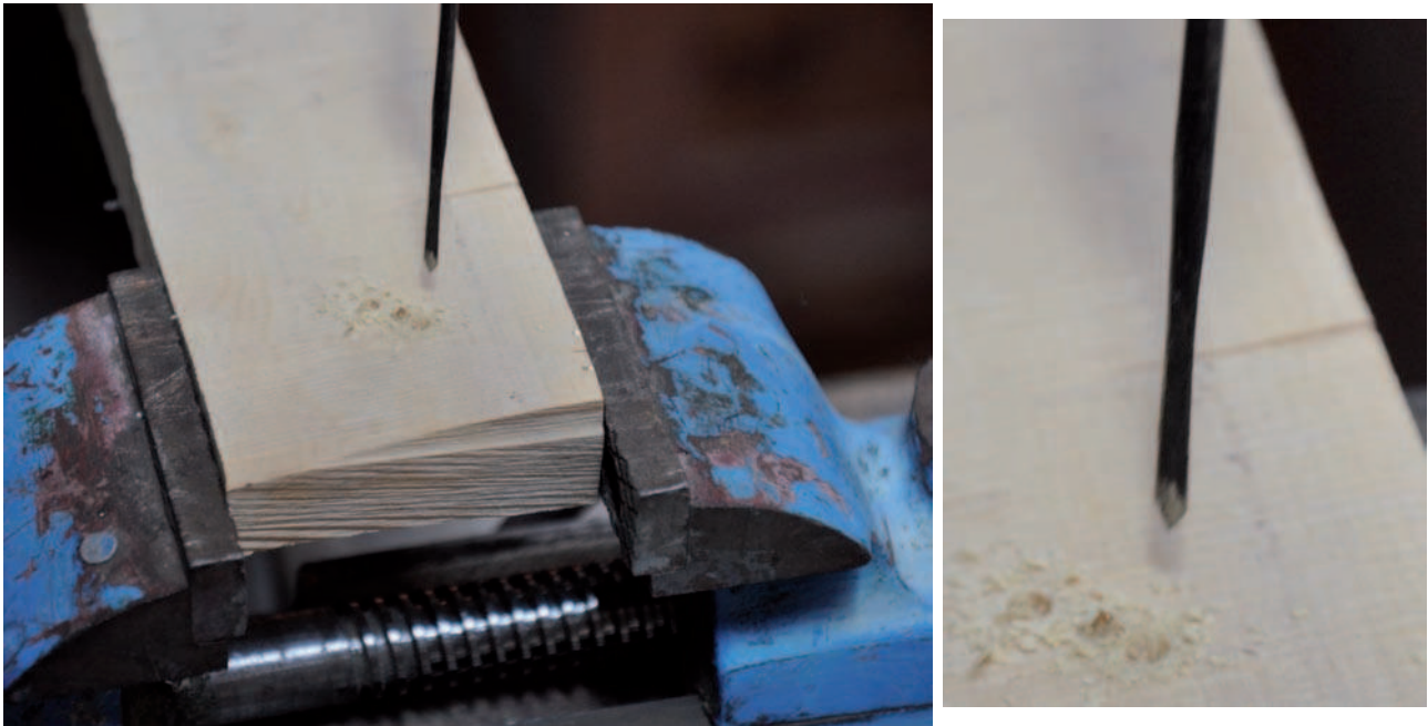
Figure 482 : Réalisation d'une simple ponctuation sur une baguette en bois, à l'aide d'une mèche à une seule pointe mise en rotation par un archet (technologie, C. Picod).
