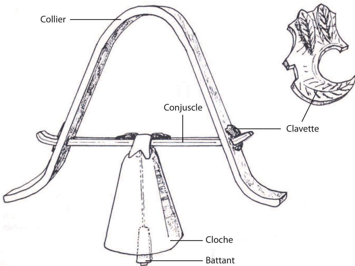
Figure 338 : Vocabulaire employé pour décrire une sonnaile (Schippers 1986, fig. 17).
