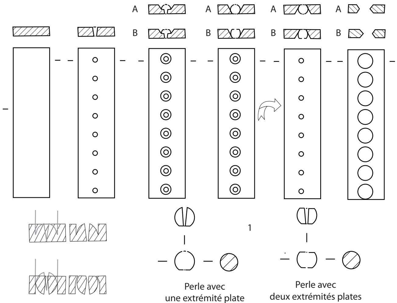
Figure 635 : Hypothèse de restitution des différentes étapes du découpage de perles à partir d'une plaquette
