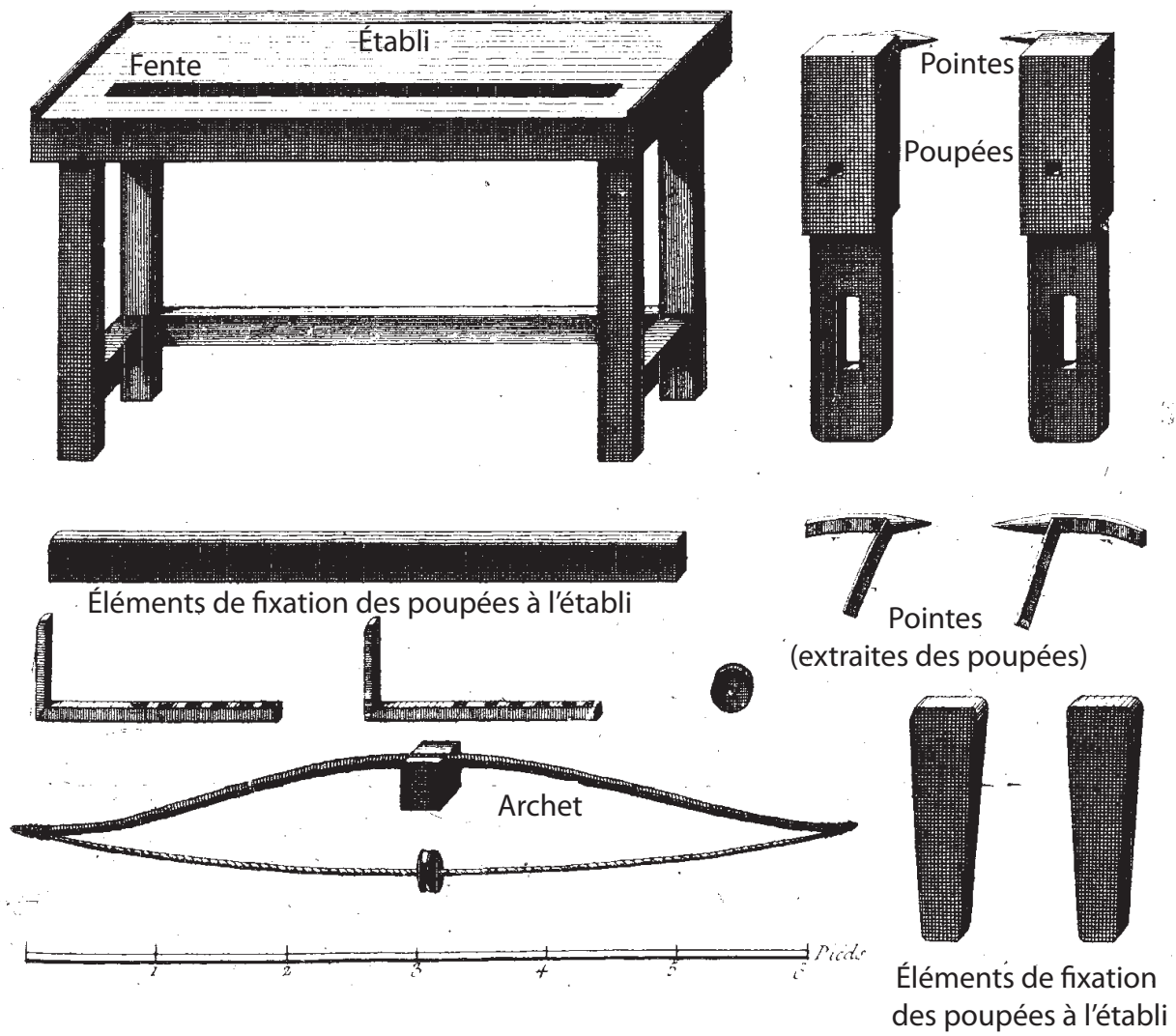
Figure 21 : L'Encyclopédie, composition d'un tour à archet, XVIII e siècle, France (Diderot et d'Alembert 1751-1777, vol. 9, pl. 2).
