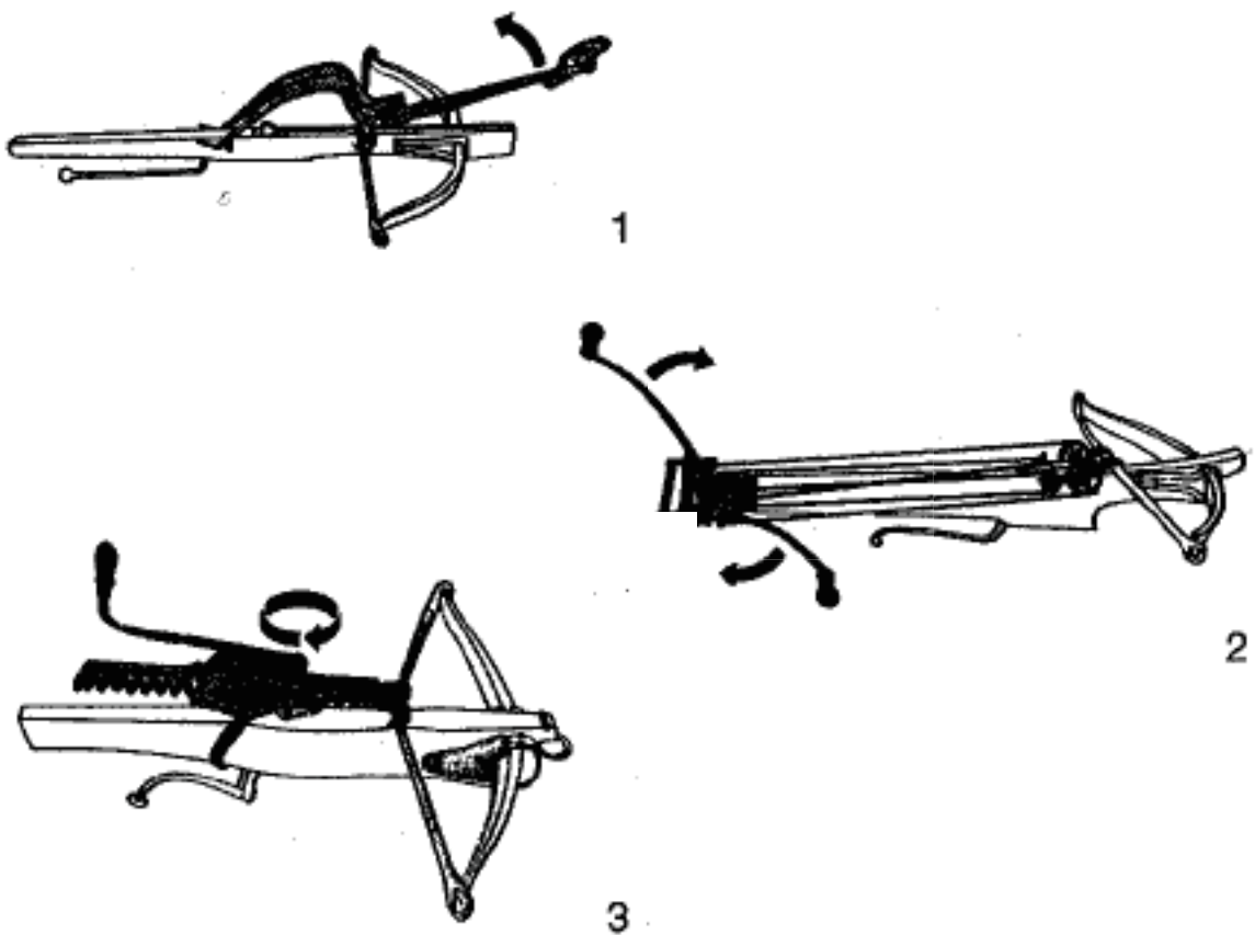
Figure 743 : Les différents mécanismes de bandage, n° 1 : pied de biche, n° 2 : tour, n° 3 : cranequin (Serdon 2005, p. 37).
