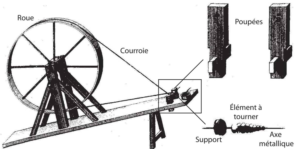
Figure 31 : L'Encyclopédie , Tour à roue et à main, XVIII e siècle, France (Diderot et d'Alembert 1751-1772, Vol. 7, section Patenôtrier, pl. II).
