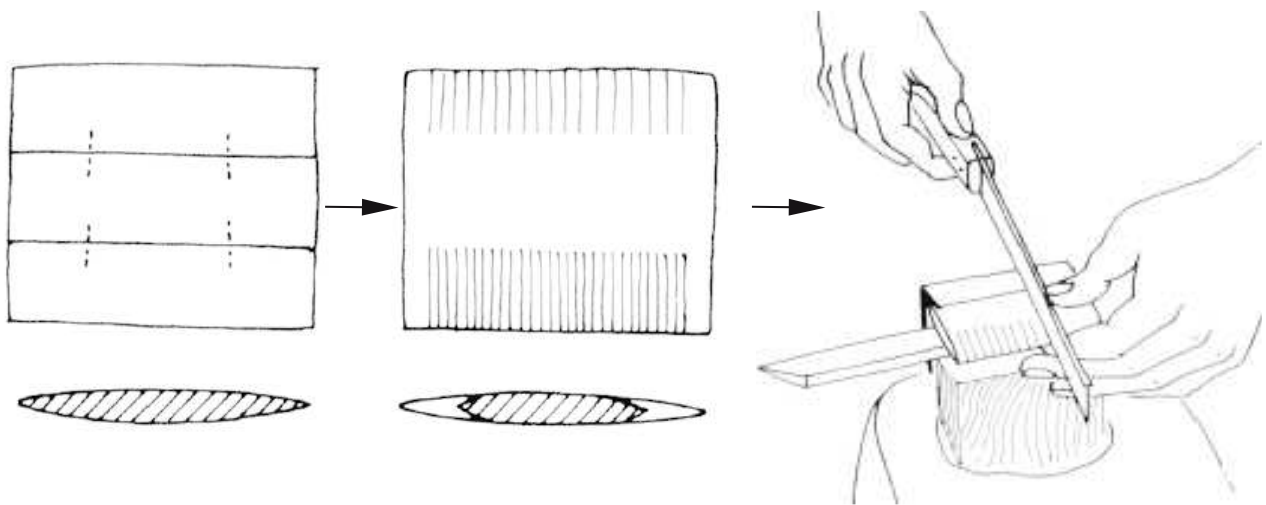
Figure 689 : Schémas proposant les différentes étapes de sciage des dents de peignes chez les artisans de Damas dans la deuxième moitié du XX e siècle, (Stordeur 1980, p. 114).
