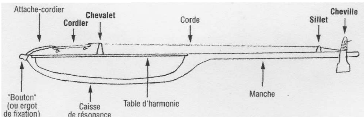
Figure 531 : Schéma d'une vièle avec la localisation d'un cordier (Homo-Lechner 1996, p. 78).
