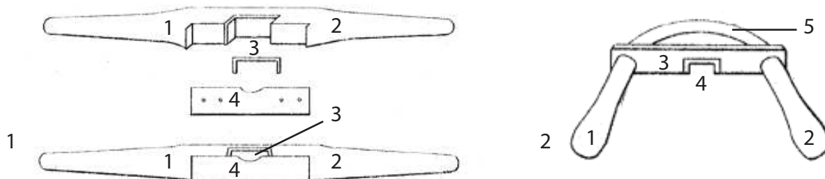
Figure 321 : Outils utilisés au XIX e siècle pour fendre les fanons de baleine (Dictionnaire technologique 1822, t. 23, pl. 7, n° 3-5).
