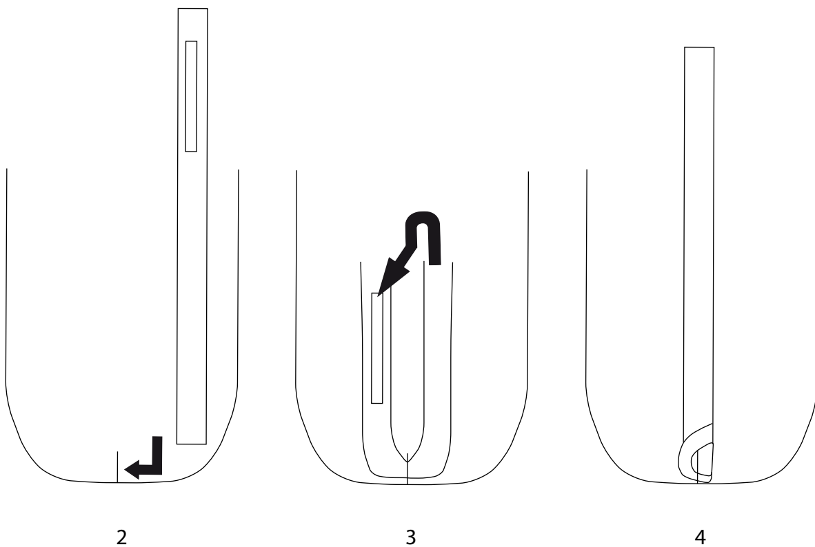
Figure 350 : Schémas présentant les différentes étapes de fixation des battants en os dans les cloches contemporaines.
