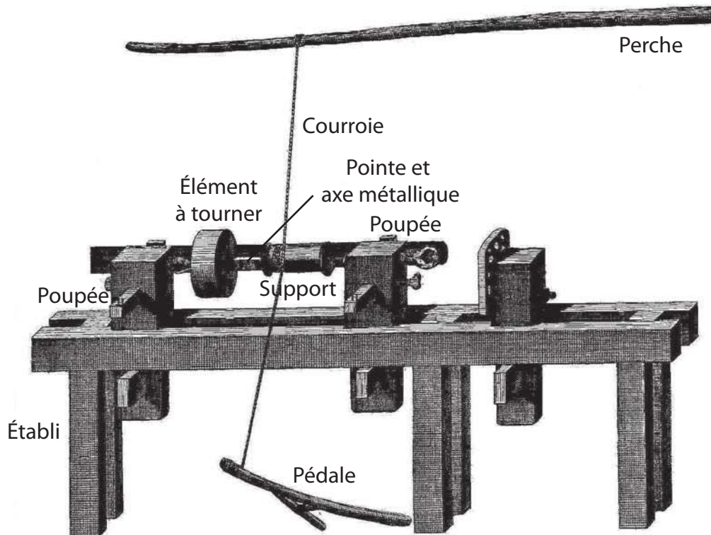
Figure 29 : L'Encyclopédie , tour à perche et à pédale, XVIII e siècle, France, (Diderot et d'Allembert 1751-1772, vol. 8, pl. XV).
