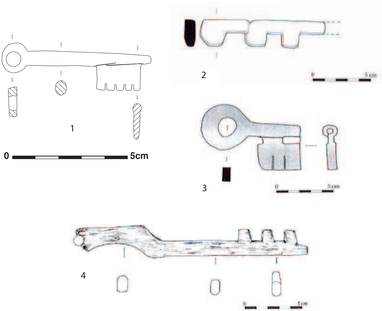
Figure 417 : n° 1, clef en bois de cervidé, n°2-3, clefs en bois (Linlaud 2014, p. 74, p. 287), n° 4, clef en métal (Linlaud 2014, p. 259, n° 12, dessin V. Aubourg).
