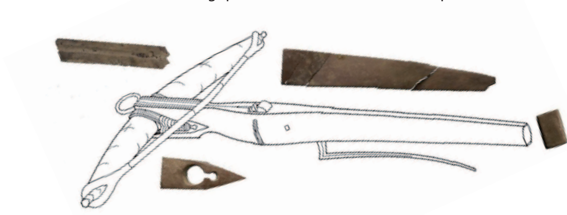
Figure 768 : Reconstitution du positionnement des plaquettes sur une arbalète, (Groote, Moens et al. n.d., n.p.).
