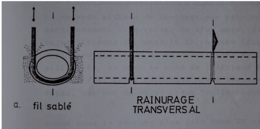
Figure 47 : Schéma présentant le technique du sciage à la ficelle, (Murray 1982, p. 88).
