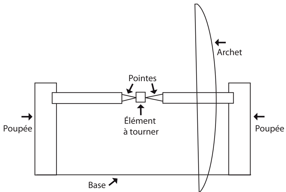
Figure 15 : Schéma de reconstitution d'un tour à archet.
