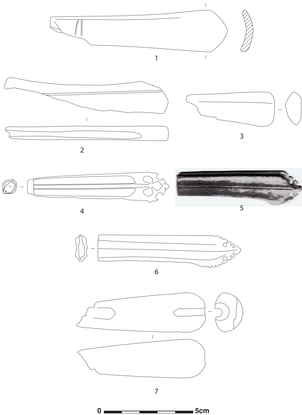
Figure 359 : Manches monoblocs en os et en ivoire provenant de couteaux à soie.
