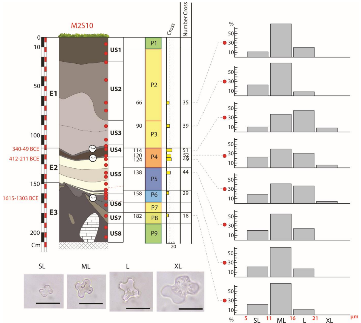
Figure 5.5 – Distribution des classes morphométriques de morphotypes Cross au sein de 8 échantillons du sondage M2S10. Le morphotype XL, supérieur à 21 µm est interpréter comme indicateur de maïs.
