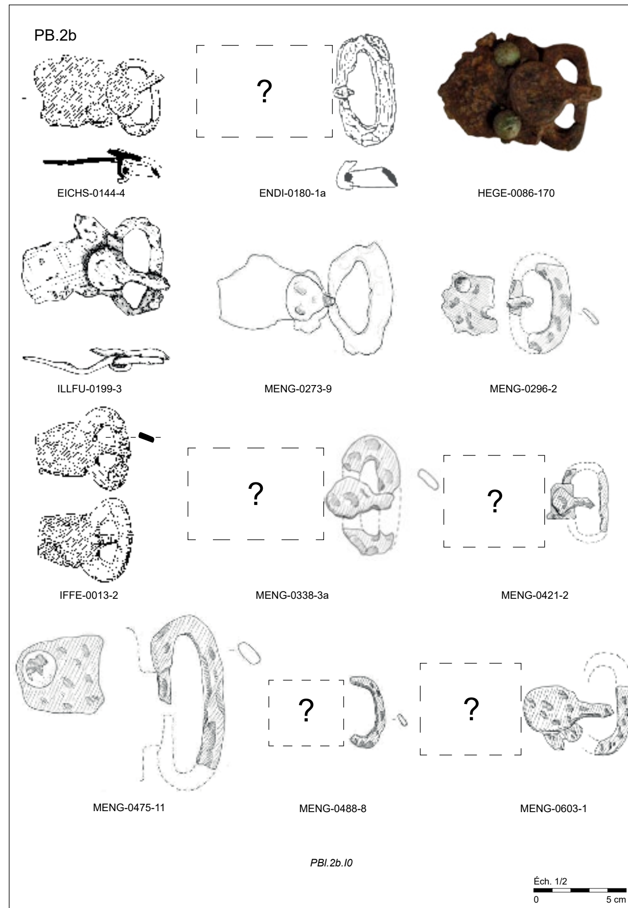
Plaques-boucles en fer non damasquiné de formes indéterminées (PB.2b.I).
