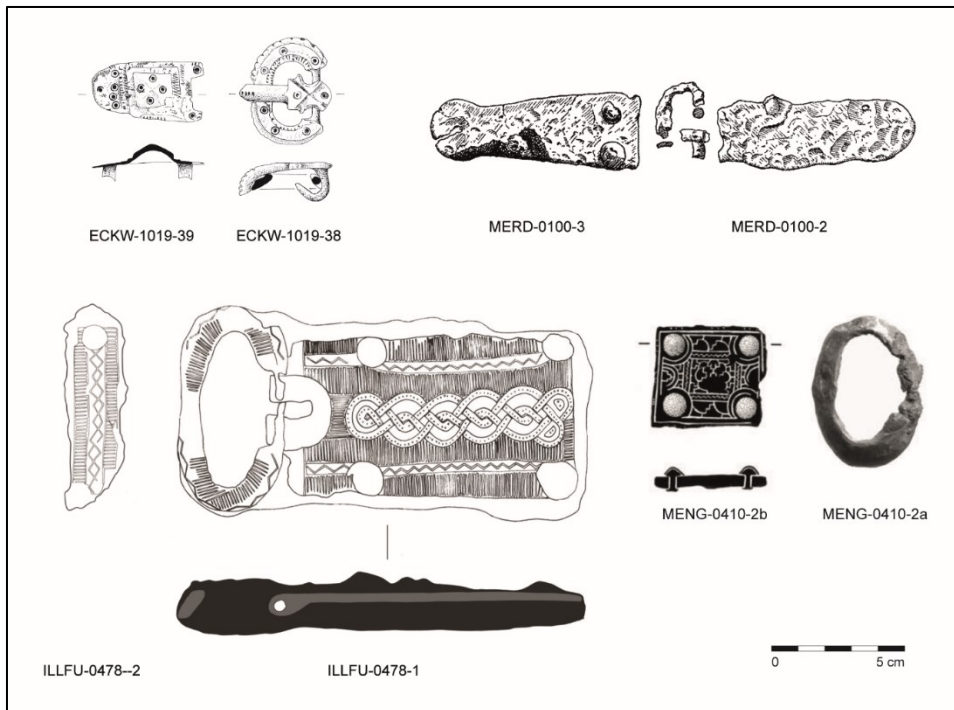
Figure 116 : Garnitures bipartites des sépultures féminines.
