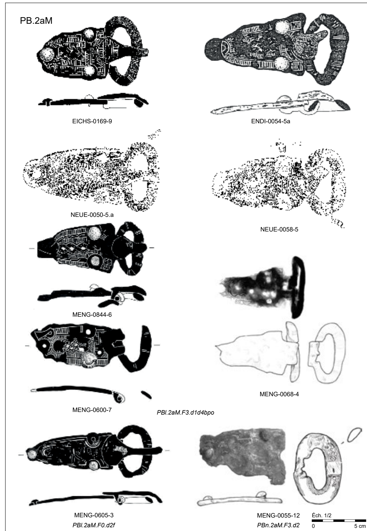
Plaques-boucles en fer damasquiné monochrome à plaques linguiformes (PB.2aM.F).
