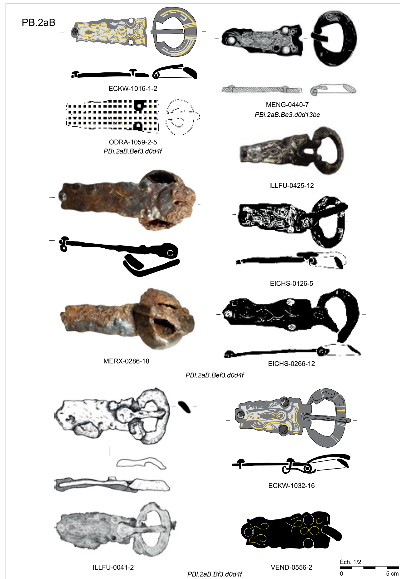
Plaques-boucles en fer damasquiné bichrome à plaques trapézoïdales (PB.2aB.B).
