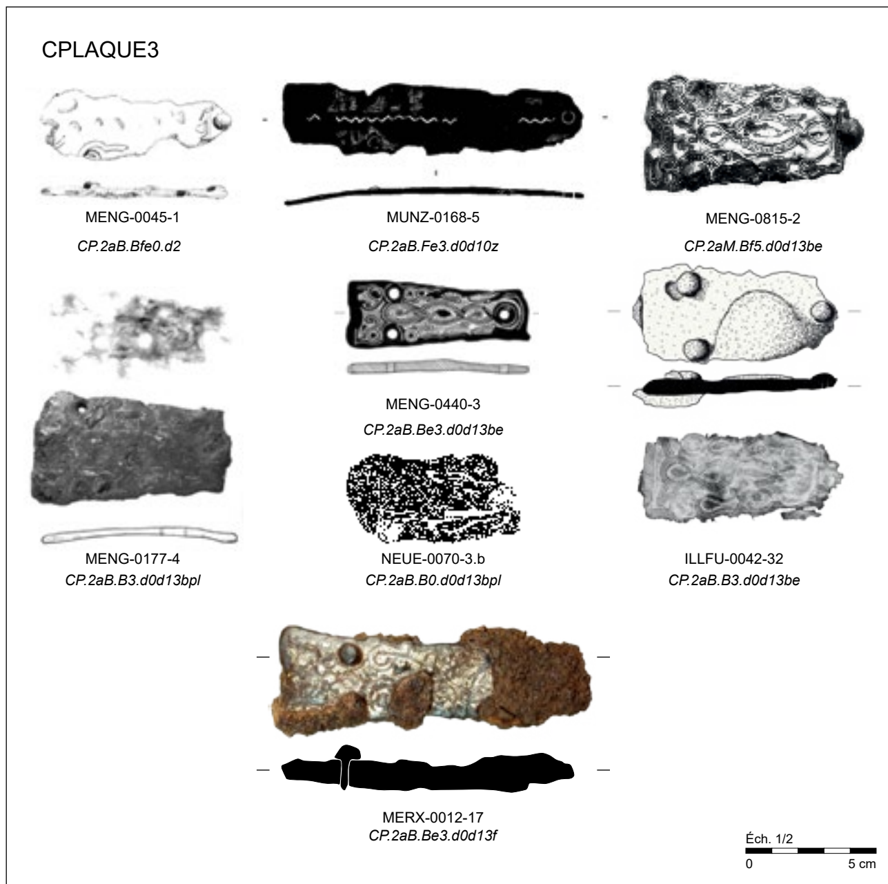
Contre-plaques du groupe typologique CPLAQUE3.
