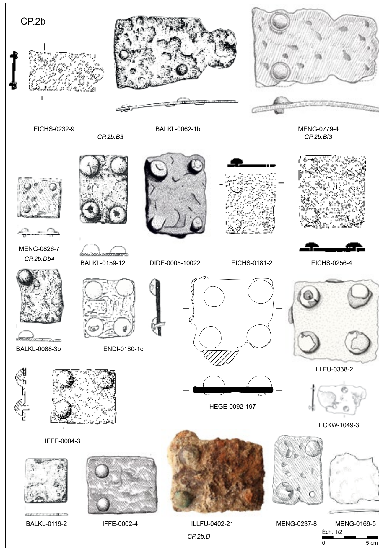
Contre-plaques en fer non damasquiné de formes trapézoïdales (CP.2b.B) et quadrangulaires (CP.2b.D).
