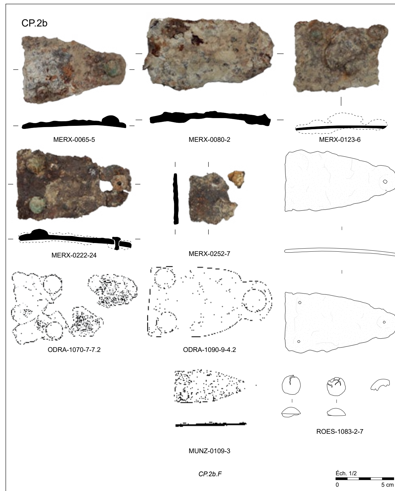
Contre-plaques en fer non damasquiné de formes linguiformes (CP.2b.F).
