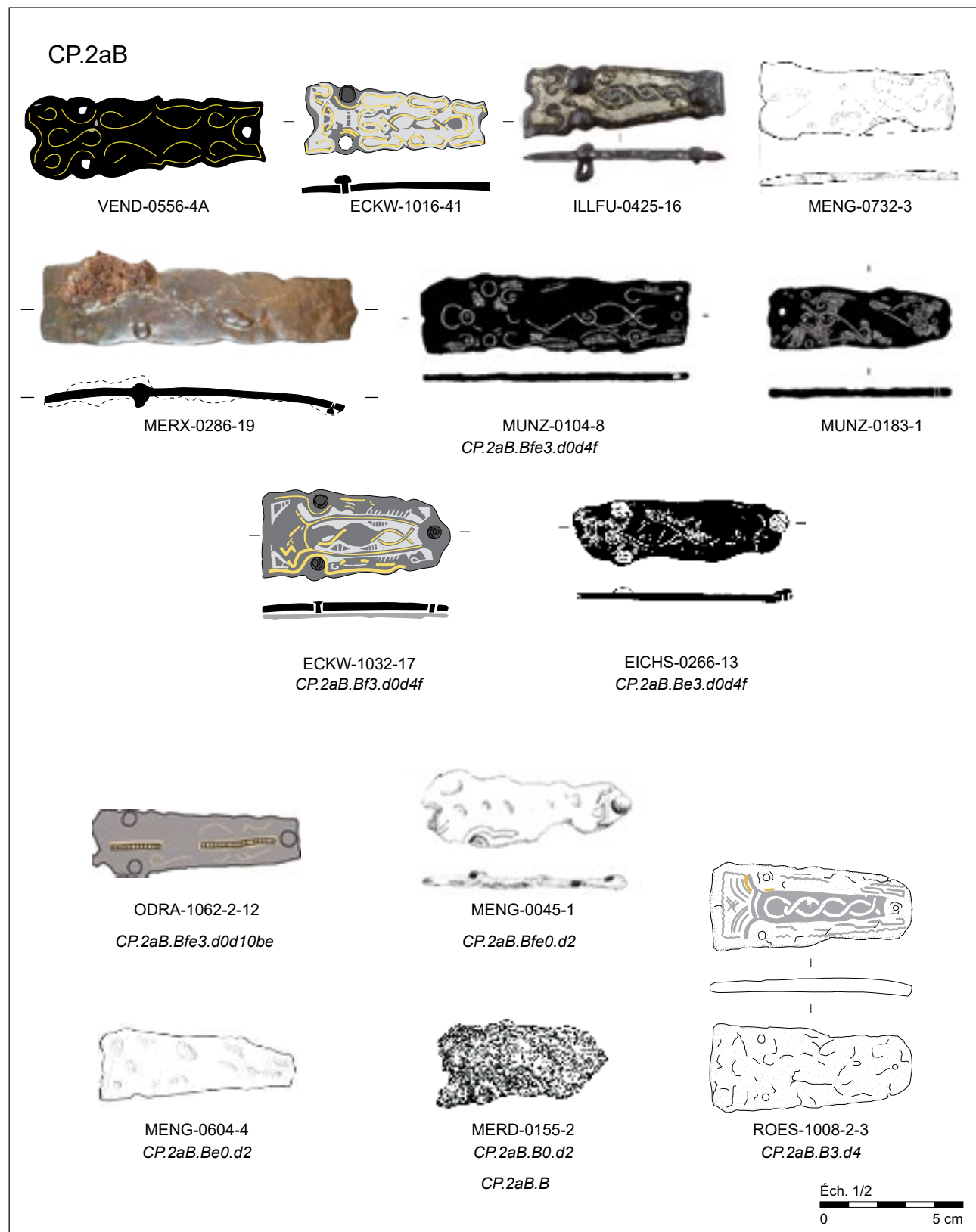
Contre-plaques en fer damasquiné bichrome de formes trapézoïdales (CP.2aB.B).
