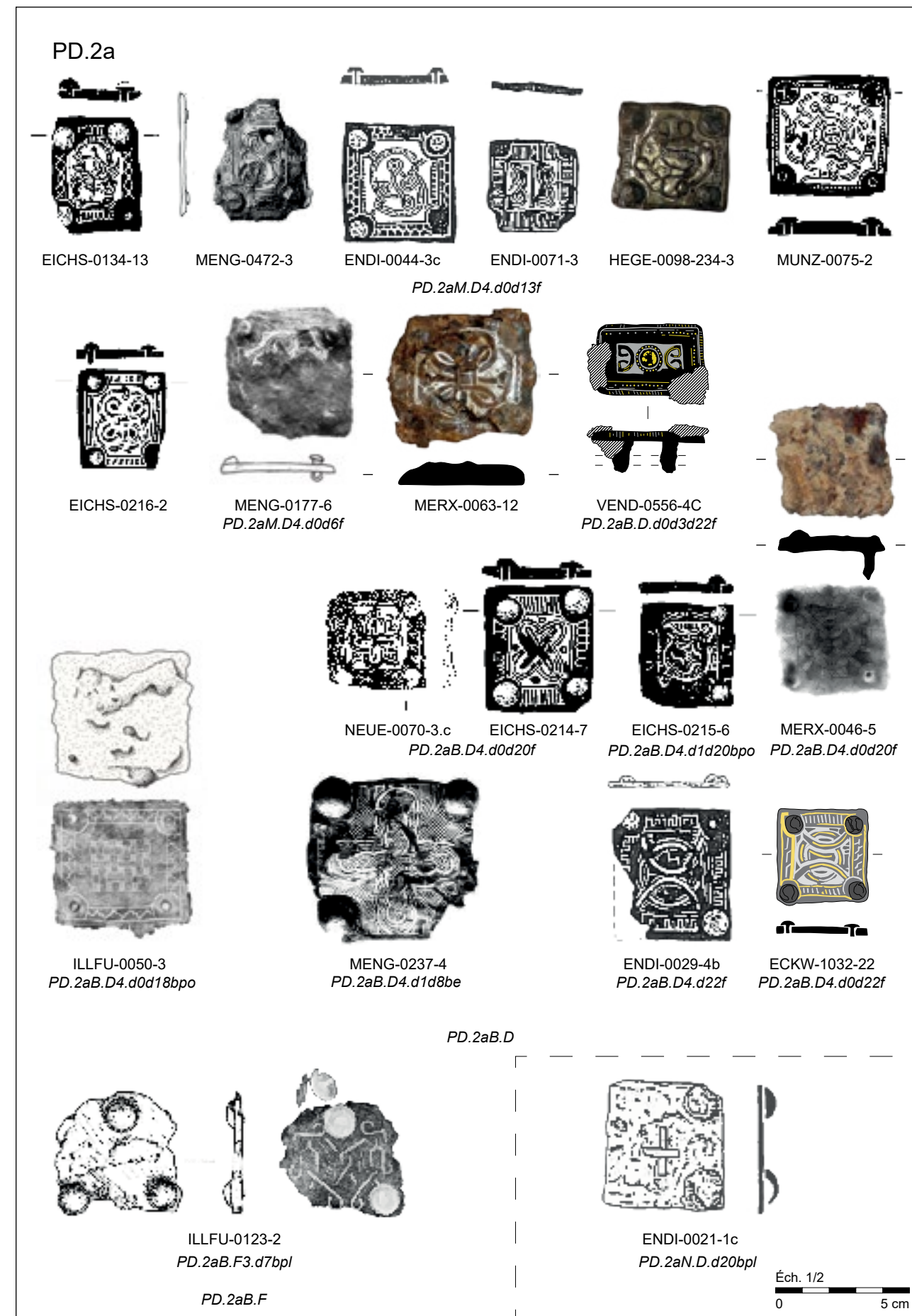
Plaques dorsales en fer damasquiné bichrome de formes quadrangulaires (PD.2aB.D) et linguiformes (PD.2aB.F) et en fer damasquiné indéterminé de forme quadrangulaire (PD.2aN.D).
