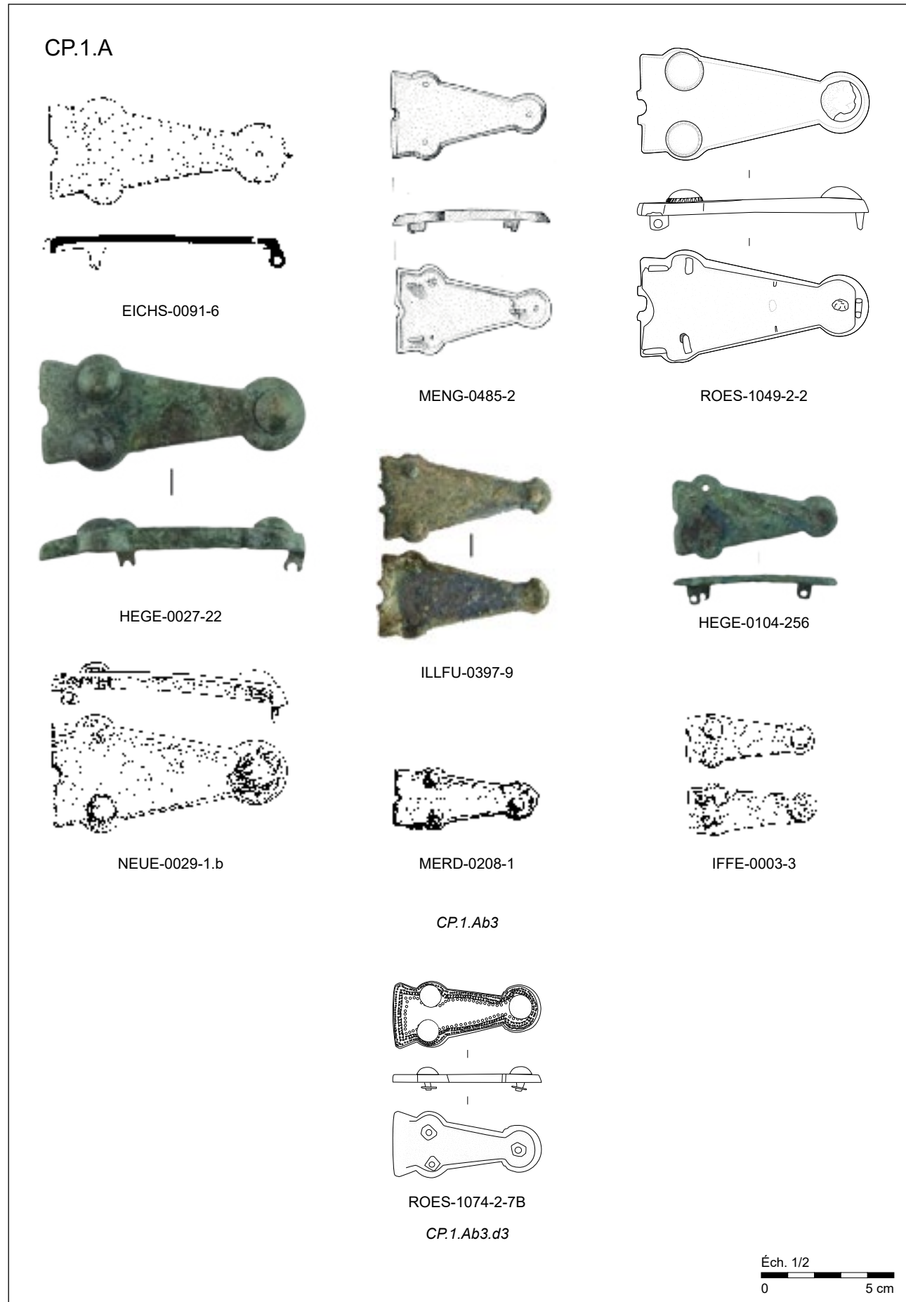
Contre-plaques en métaux non ferreux de formes triangulaires (CP.1.A).
