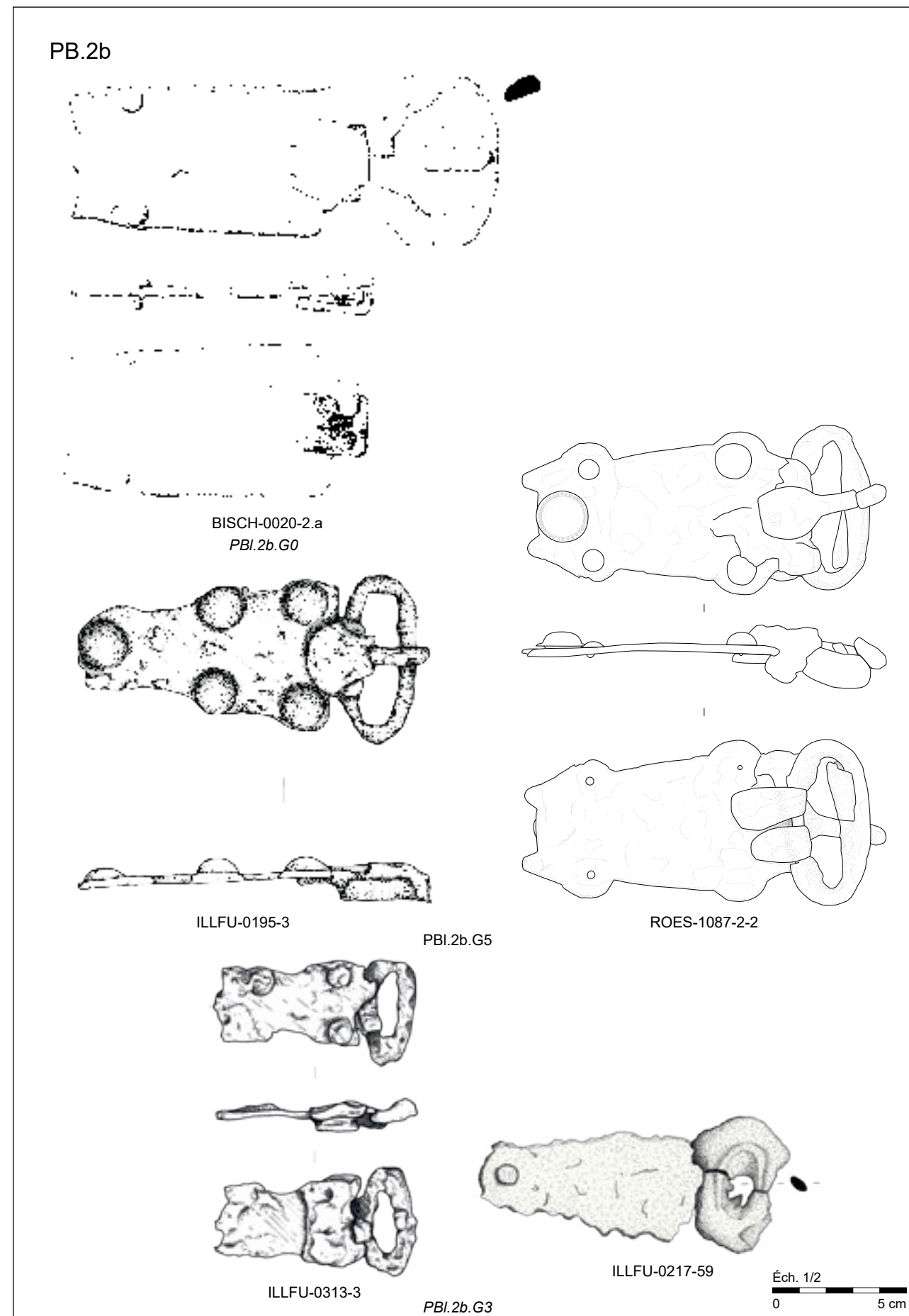
Plaques-boucles en fer non damasquiné à plaques trapézoïdales à extrémités en queues-d'arondes (PB.2b.G).
