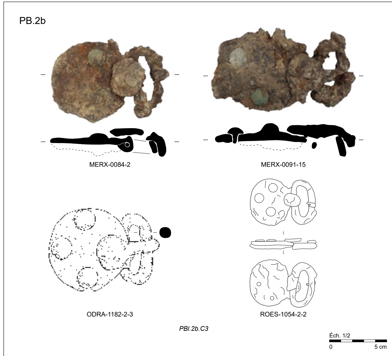
Plaques-boucles en fer non damasquiné à plaques rondes (PB.2b.C).
