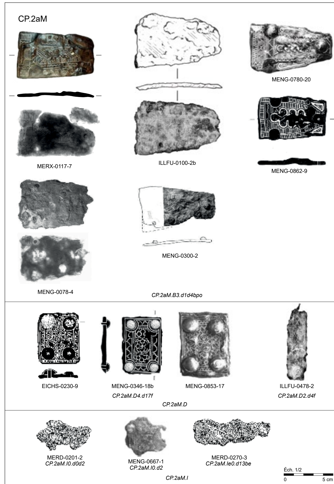
Contre-plaques en fer damasquiné monochrome de formes trapézoïdales (CP.2aM.B), quadrangulaires (CP.2aM.D) et indéterminées (CP.2aM.I).
