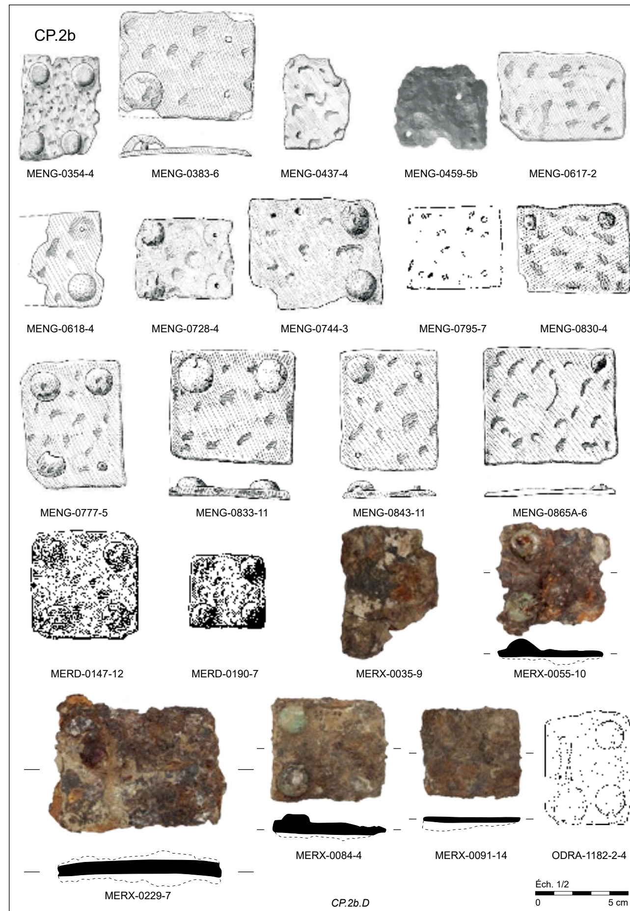
Contre-plaques en fer non damasquiné de formes quadrangulaires (CP.2b.D).
