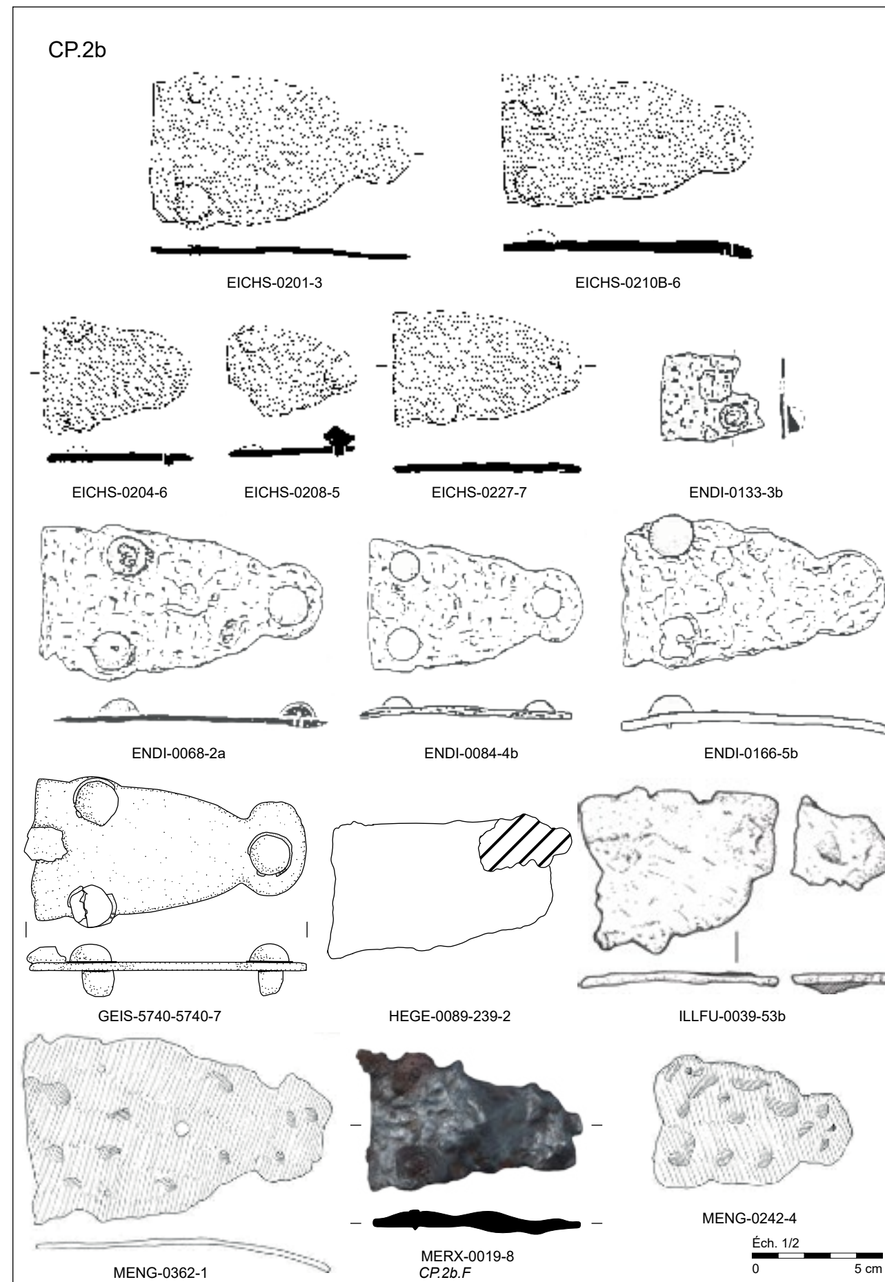
Contre-plaques en fer non damasquiné de formes linguiformes (CP.2b.F).
