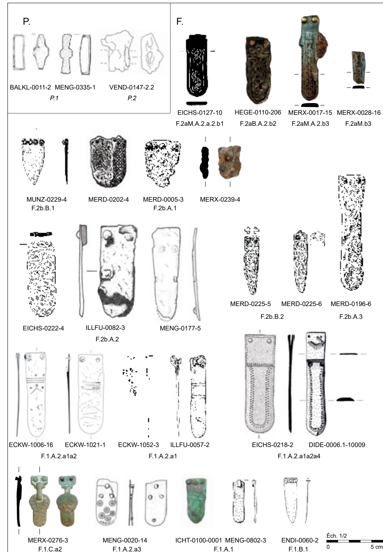
Passants en métaux non ferreux (P.1) et en fer non damasquiné (P.2), ferrets moyens et courts en fer damasquiné monochrome (F.2aM) et bichrome (F.2aB), en fer non damasquiné (F.2b) et en métaux non ferreux (F.1).
