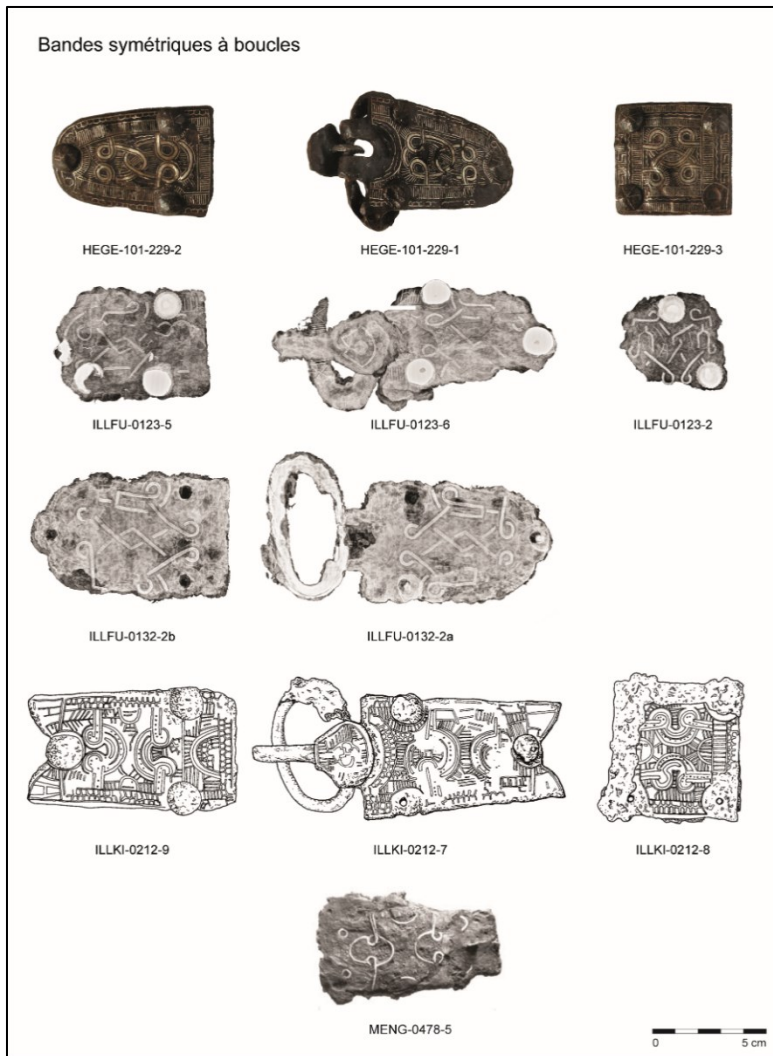
Figure 87 : Garnitures à bandes symétriques à boucles en fer damasqué.
