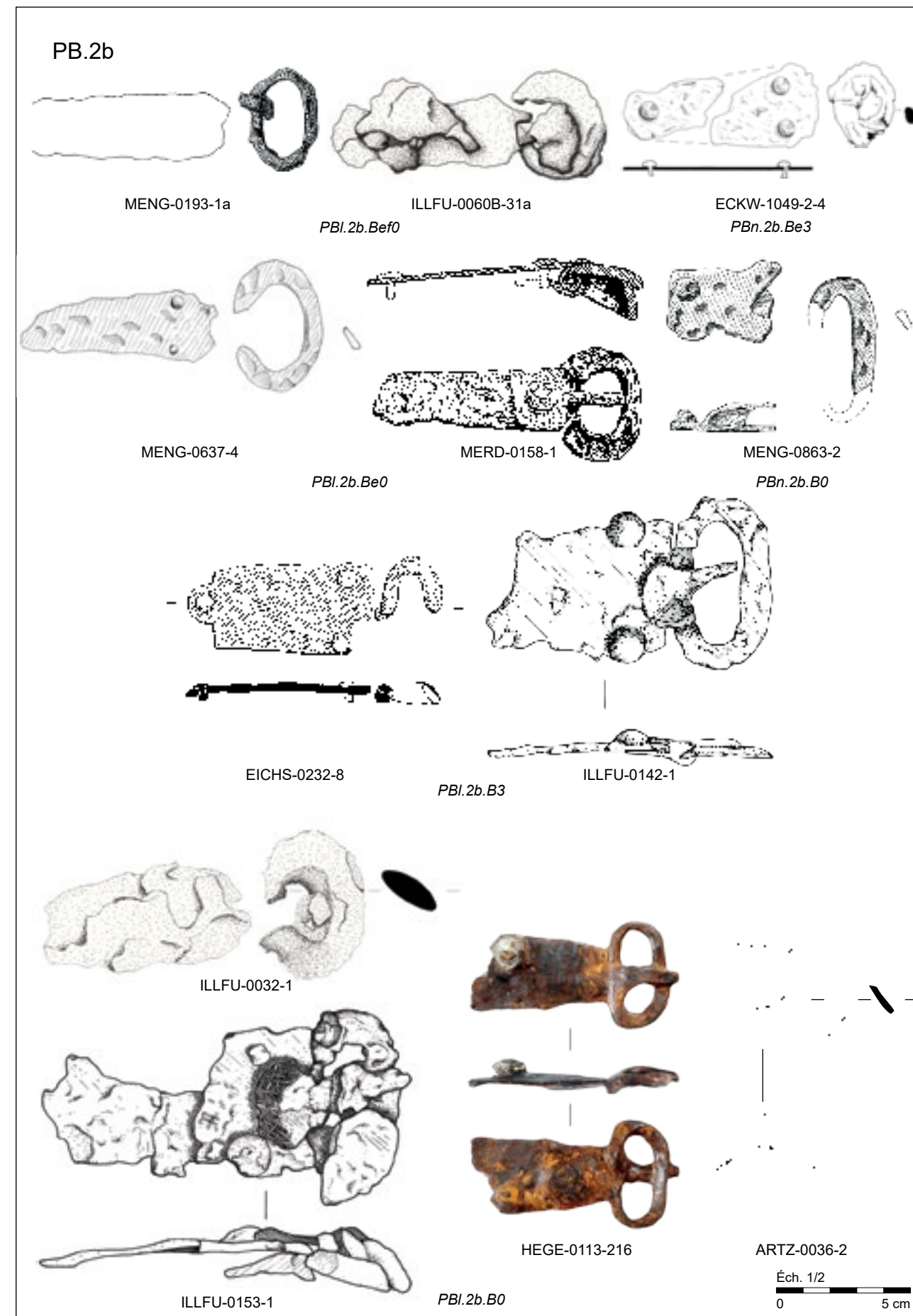
Plaques-boucles en fer non damasquiné à plaques trapézoïdales (PB.2b.B).
