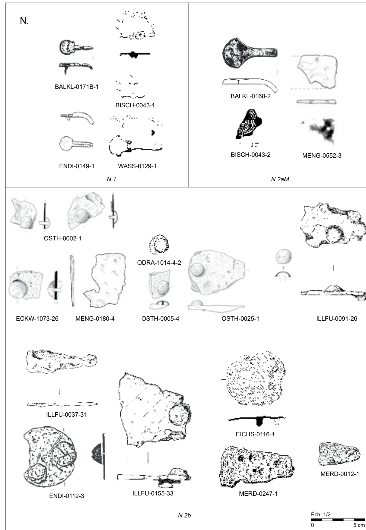
Garnitures de types indéterminés en métaux non ferreux (N.1), en fer damasquiné monochrome (N.2aM) et en fer non damasquiné (N.2b).
