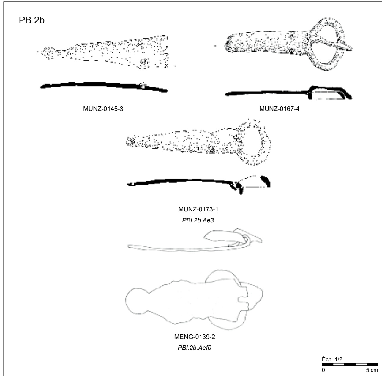
Plaques-boucles en fer non damasquiné à plaques triangulaires étroites (PB.2b.Ae) et étroites à contours festonnés (PB.2b.Aef).
