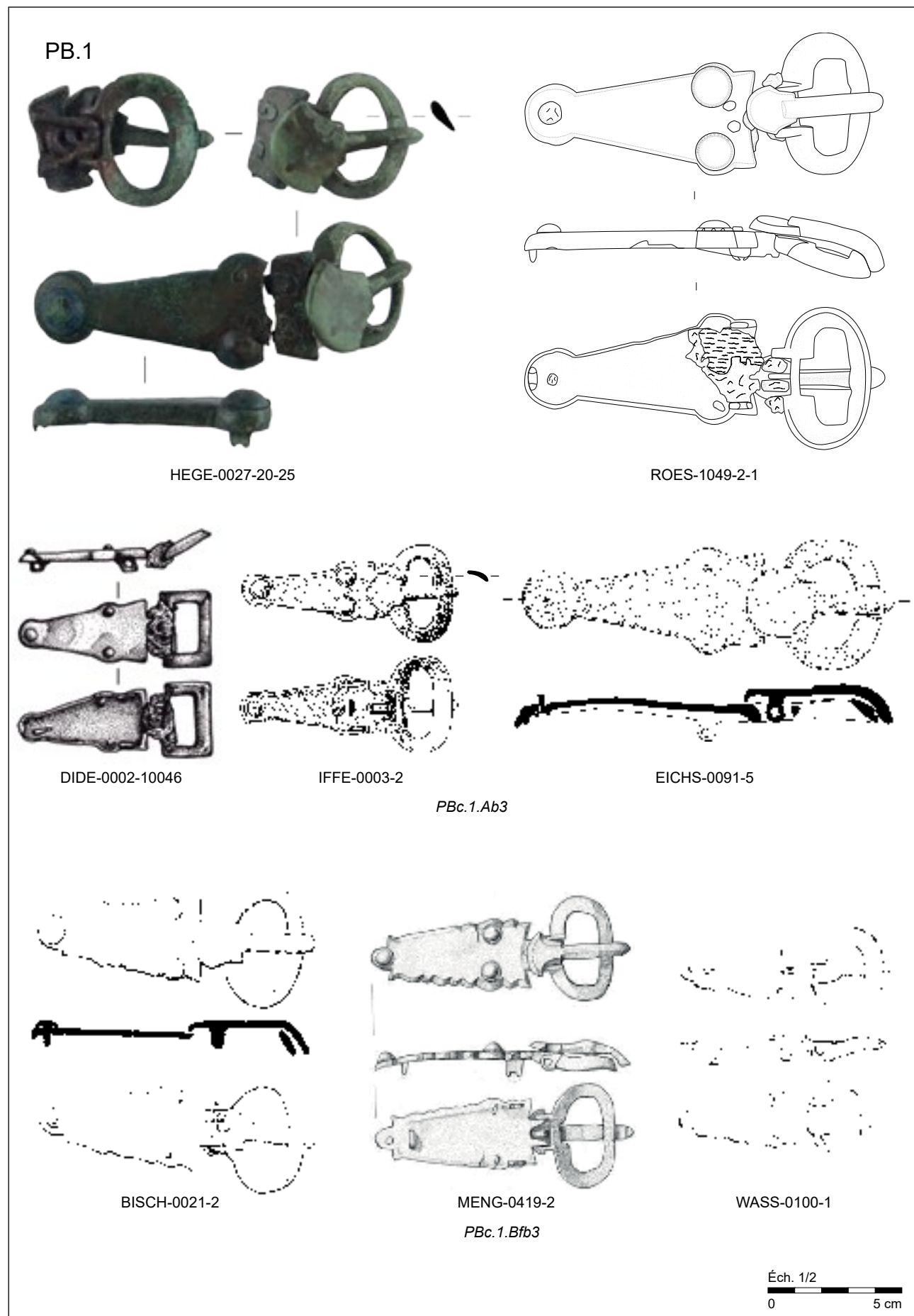
Plaques-boucles en métaux non ferreux à charnières à plaques triangulaires à bords biseautés (PBc.1.A) et trapézoïdales à contours festonnés et bords biseautés (PBc.1.Bfb).
