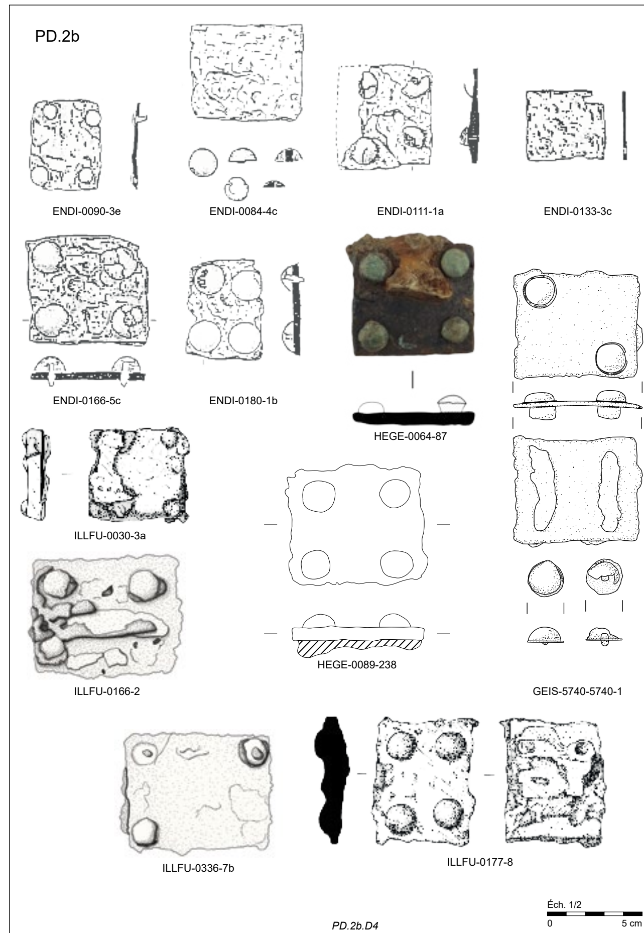
Plaques dorsales en fer non damasquiné à plaques quadrangulaires (PD.2b.D).
