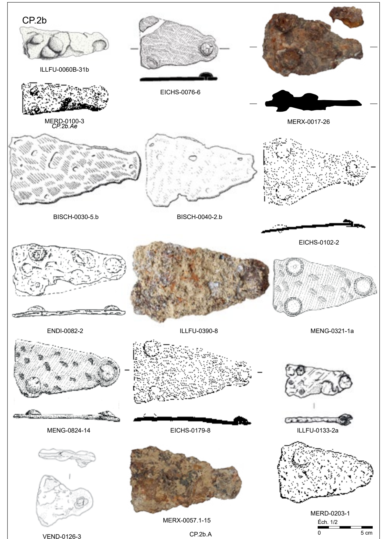
Contre-plaques en fer non damasquiné de formes triangulaires (CP.2b.A).
