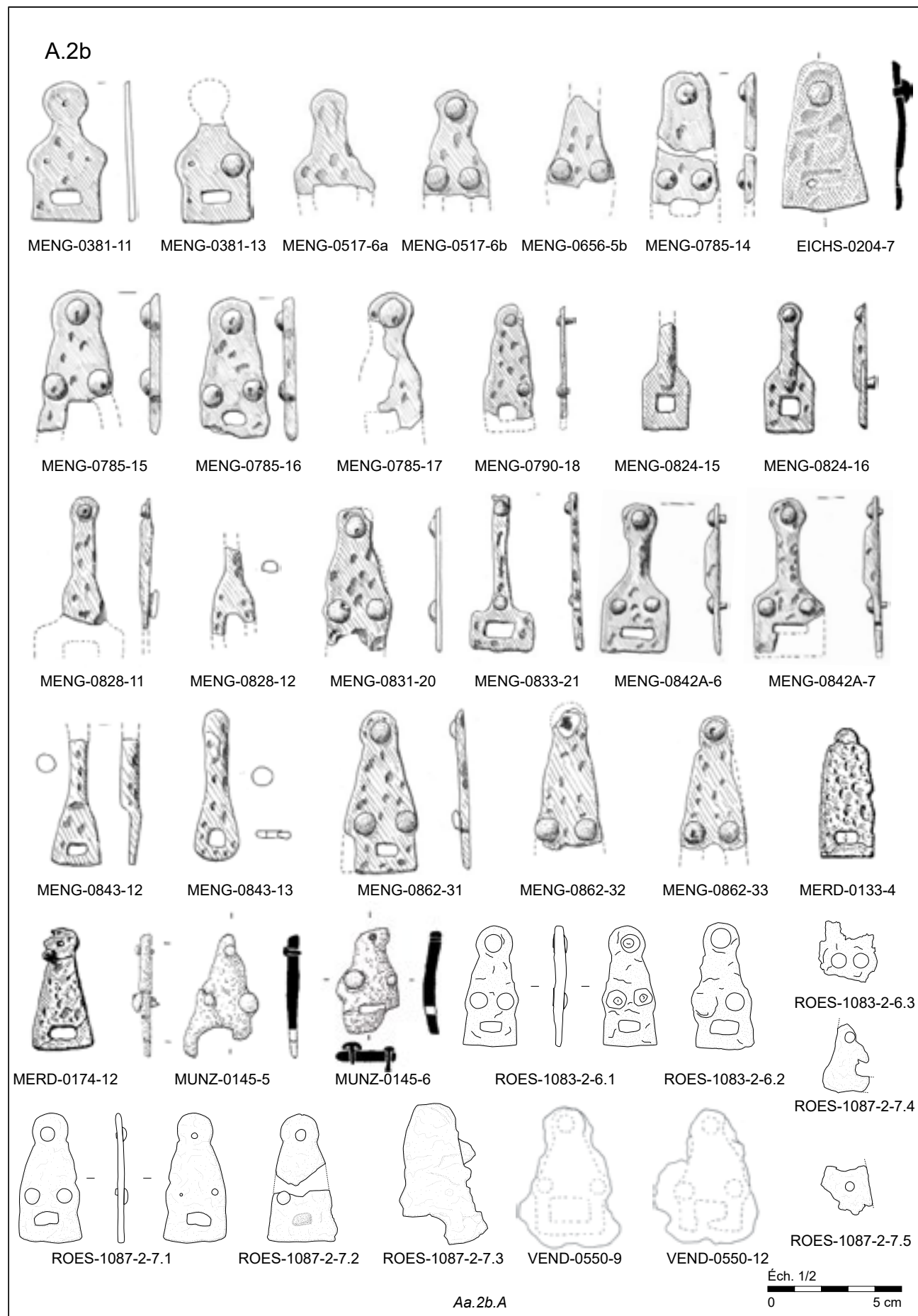
Appliques ajourées en fer non damasquiné triangulaires (Aa.2b.A).
