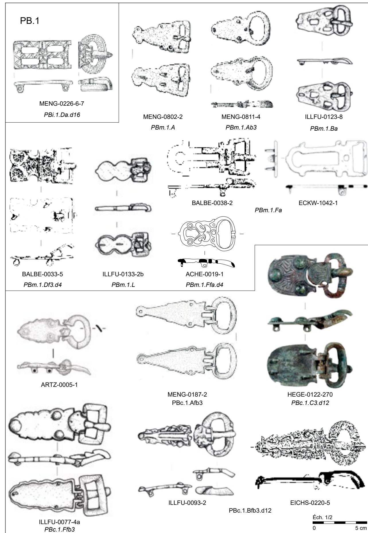
Plaques-boucles en métaux non ferreux monoblocs (PBI.1), à plaques et boucles indépendantes (PBI.1) et à charnières (PBI.1).
