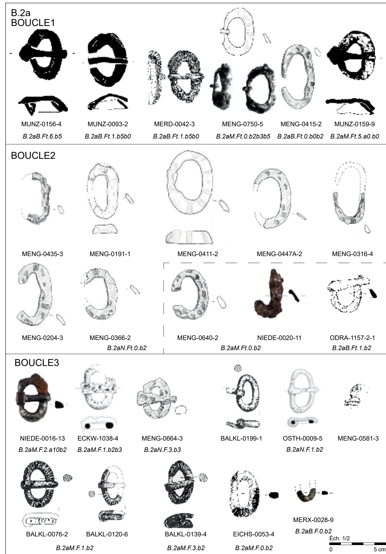
Boucles simples en fer damasquiné des groupes typologiques BOUCLE1, 2 et 3.
