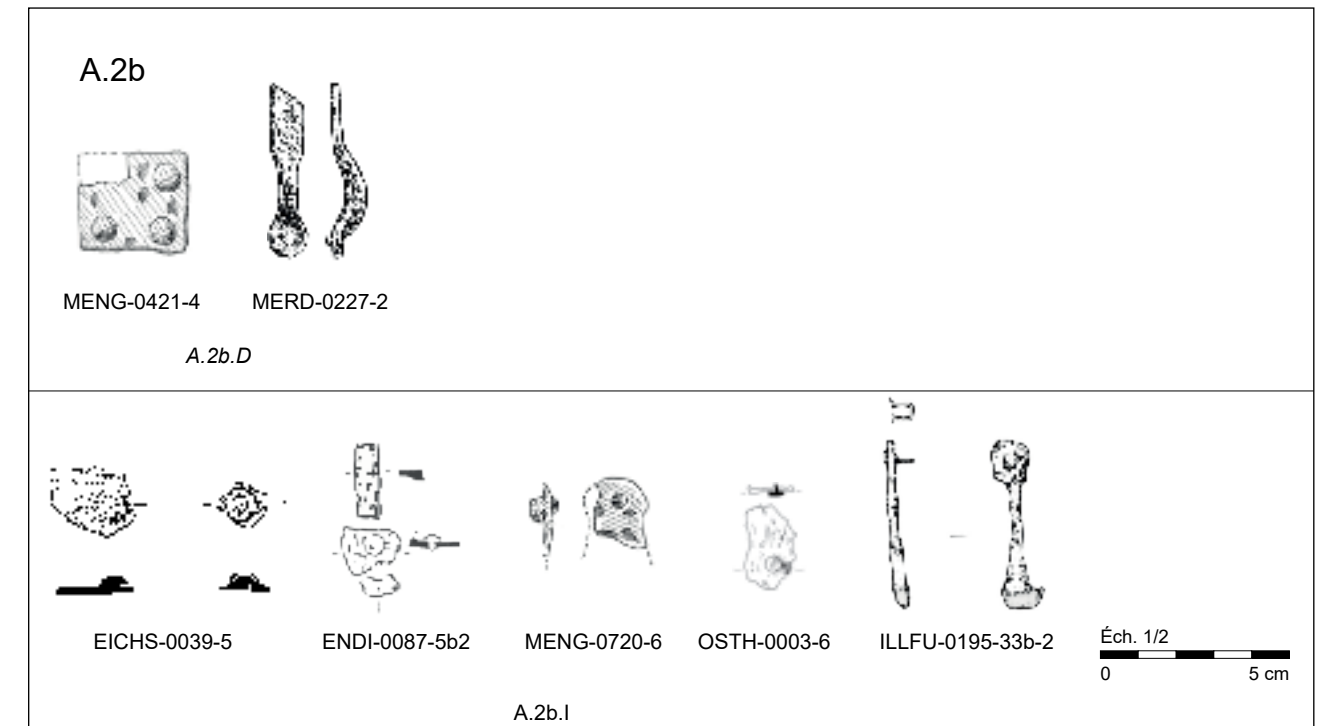
Appliques pleines en fer non damasquiné quadrangulaires (A.2b.D) et appliques de formes indéterminées (A.2b.I).
