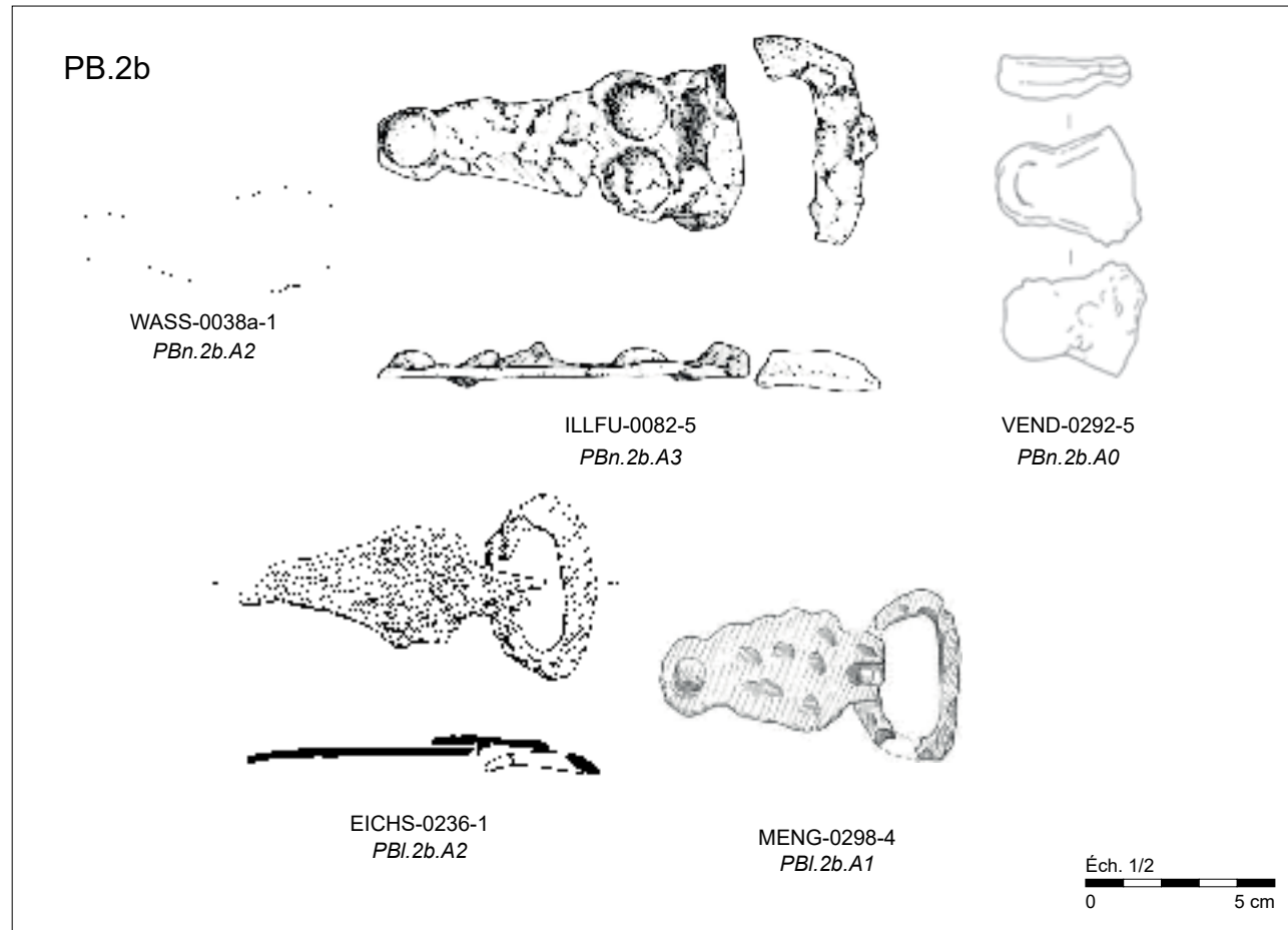
Plaques-boucles en fer non damasquiné à plaques triangulaires (PB.2b.A).
