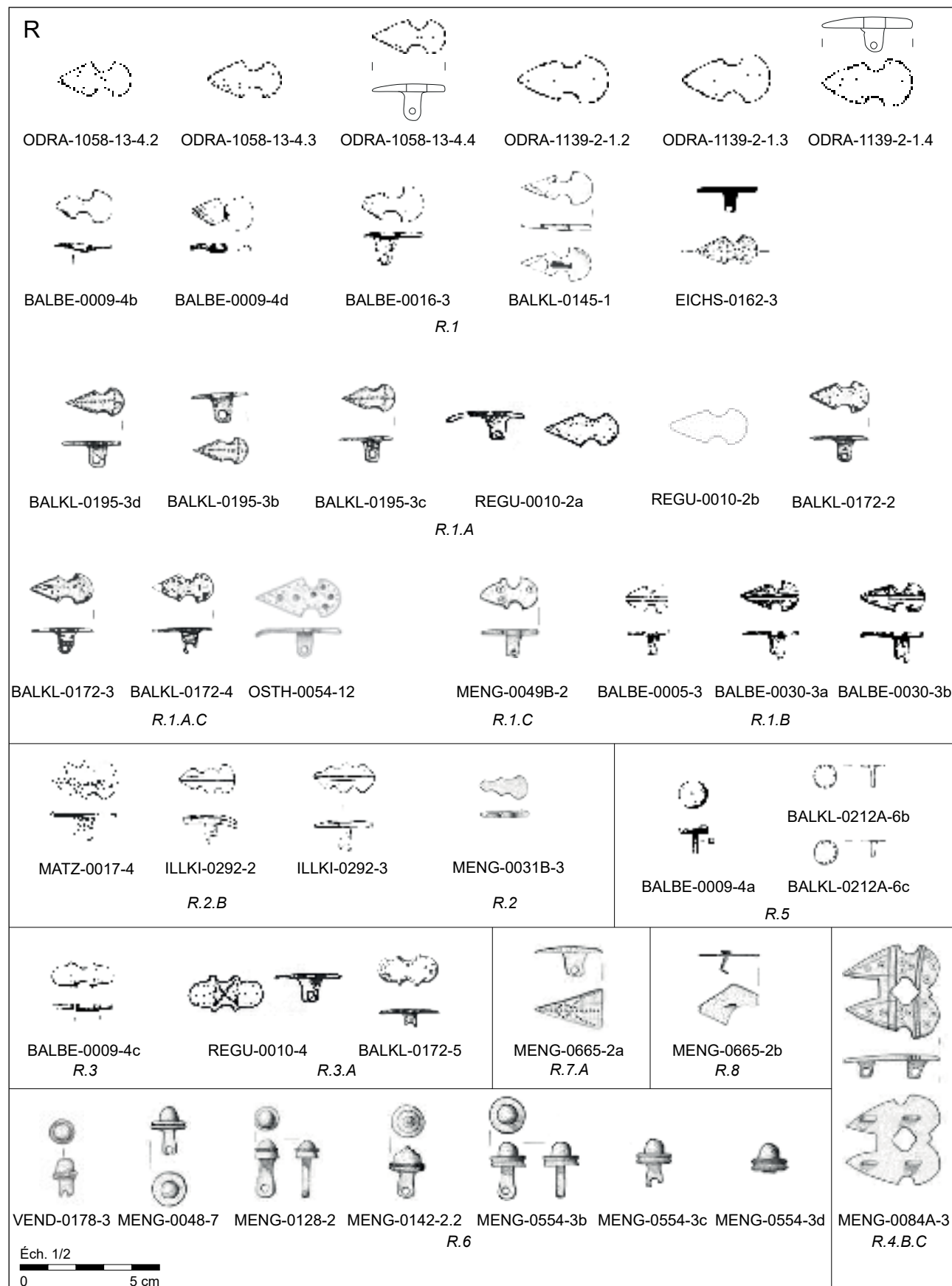
Rivets de ceintures en métaux non ferreux scutiformes à simples échancrures (R.1), doubles échancrures (R.2), scutiformes symétriques (R.3), scutiformes doubles (R.4), ronds plats (R.5), ronds hémisphériques (R.6), triangulaires (R.7) et losangiques (R.8).
