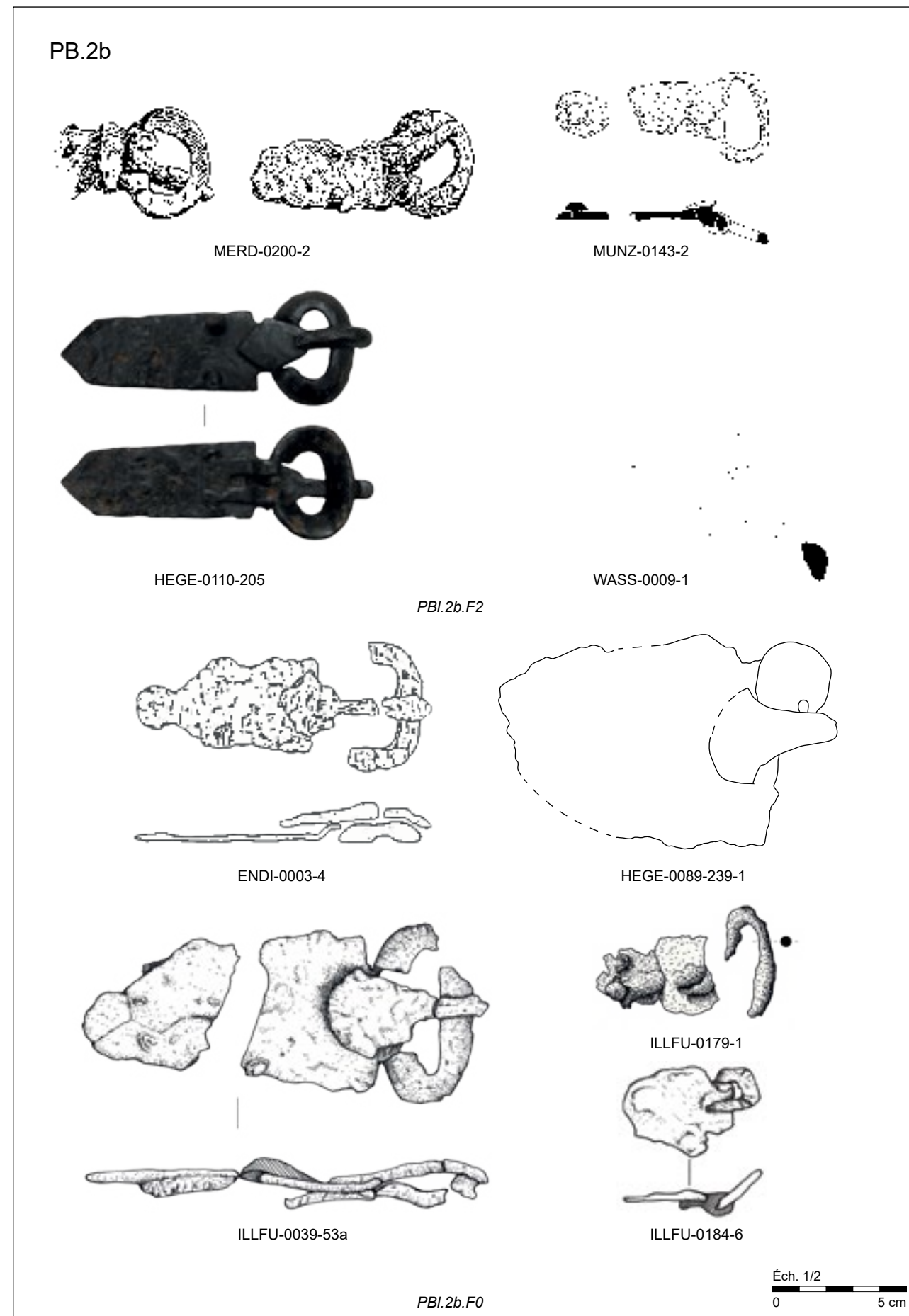
Plaques-boucles en fer non damasquiné à plaques linguiformes (PB.2b.F).
