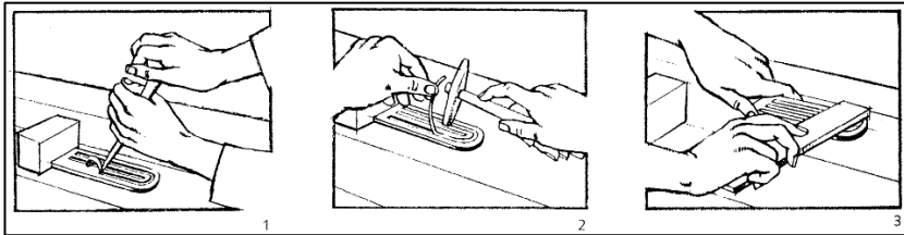
Figure 8 : La damasquinure : 1. Creusement du décor dans le fer ; 2. Incrustation d'un fil ou d'un placage ; 3. Polissage de la surface (Amrein et Binder 1996, p. 364).
