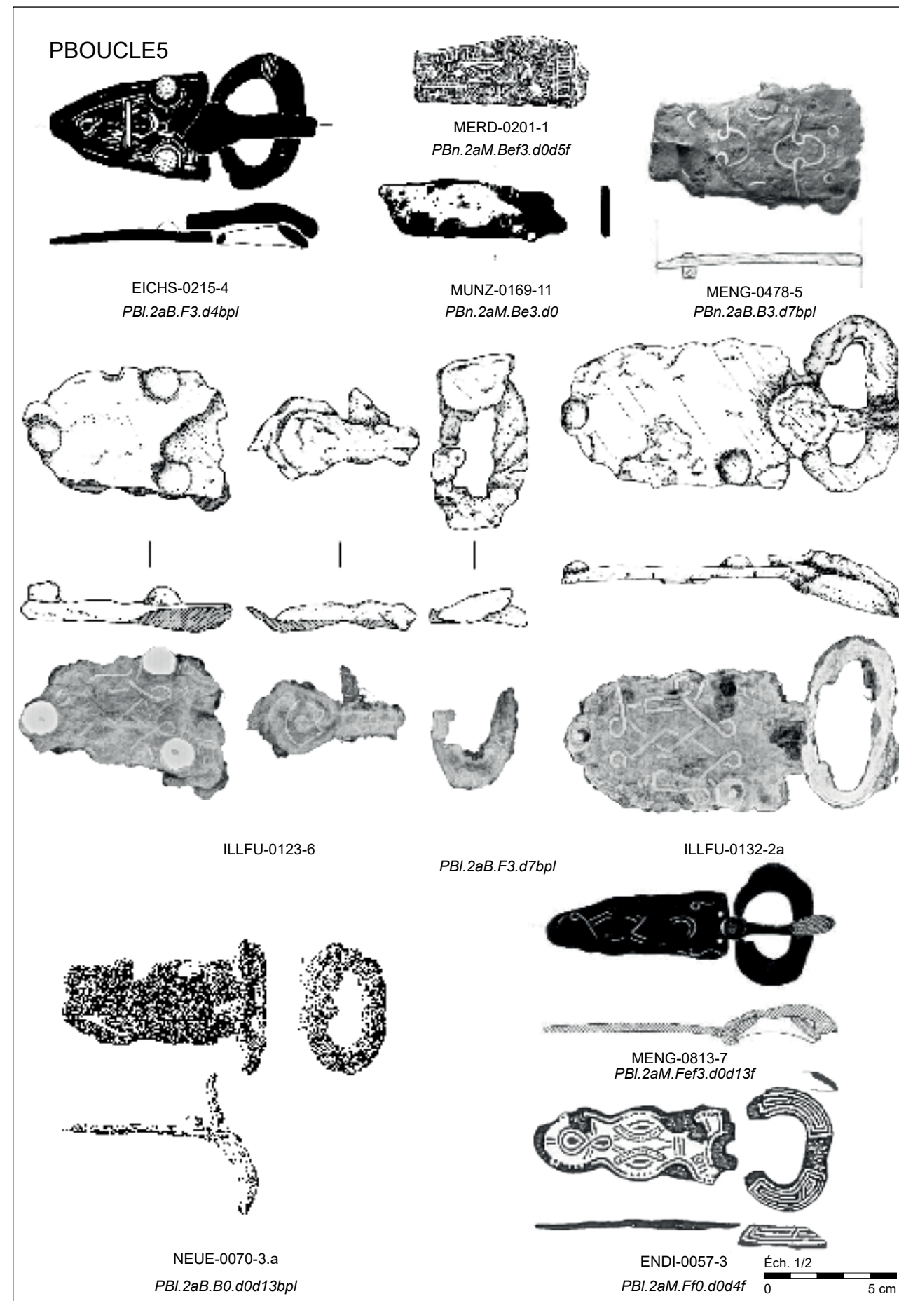
Plaques-boucles du groupe typologique PBOUCLE5.
