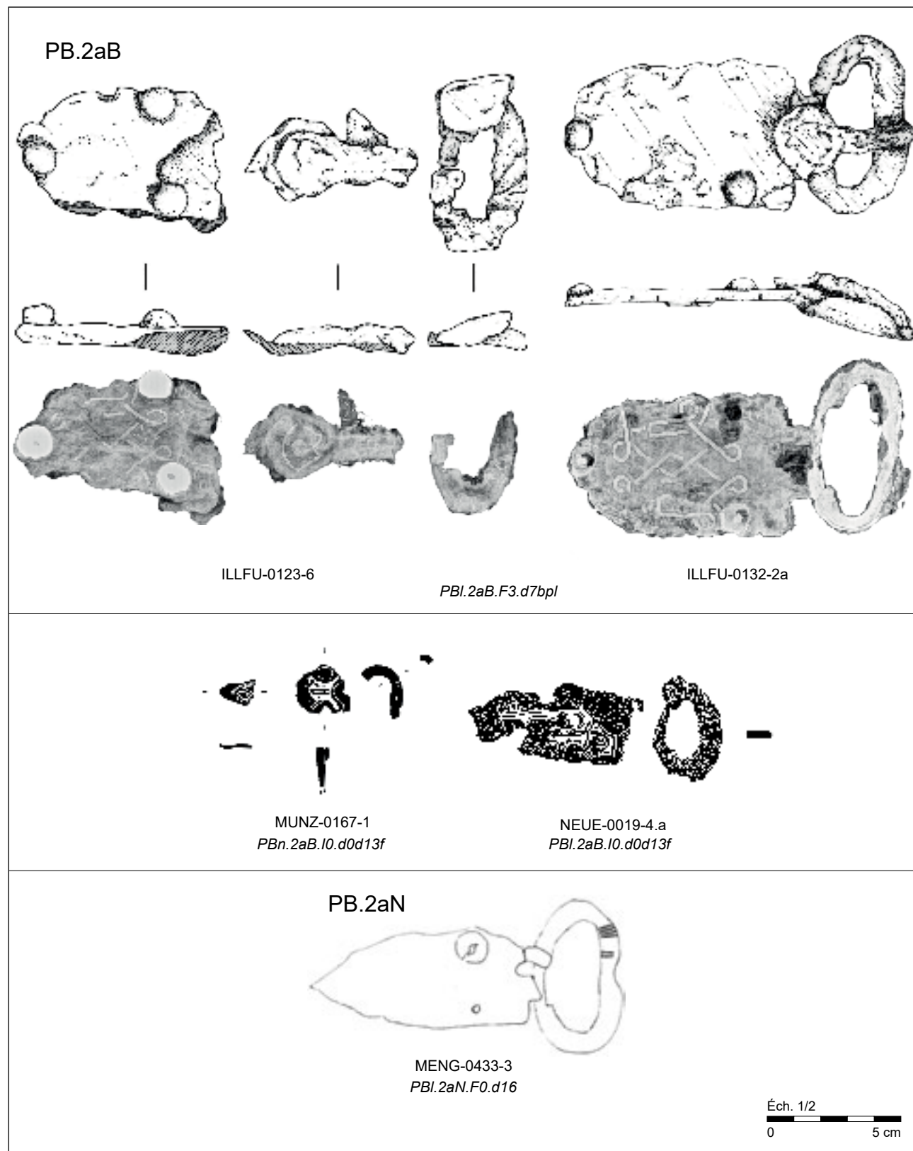
Plaques-boucles en fer damasquiné bichrome à plaques linguiformes (PB.2aB.F) et indéterminées (PB.2aB.I) et en fer damasquiné indéterminé (PB.2aN).
