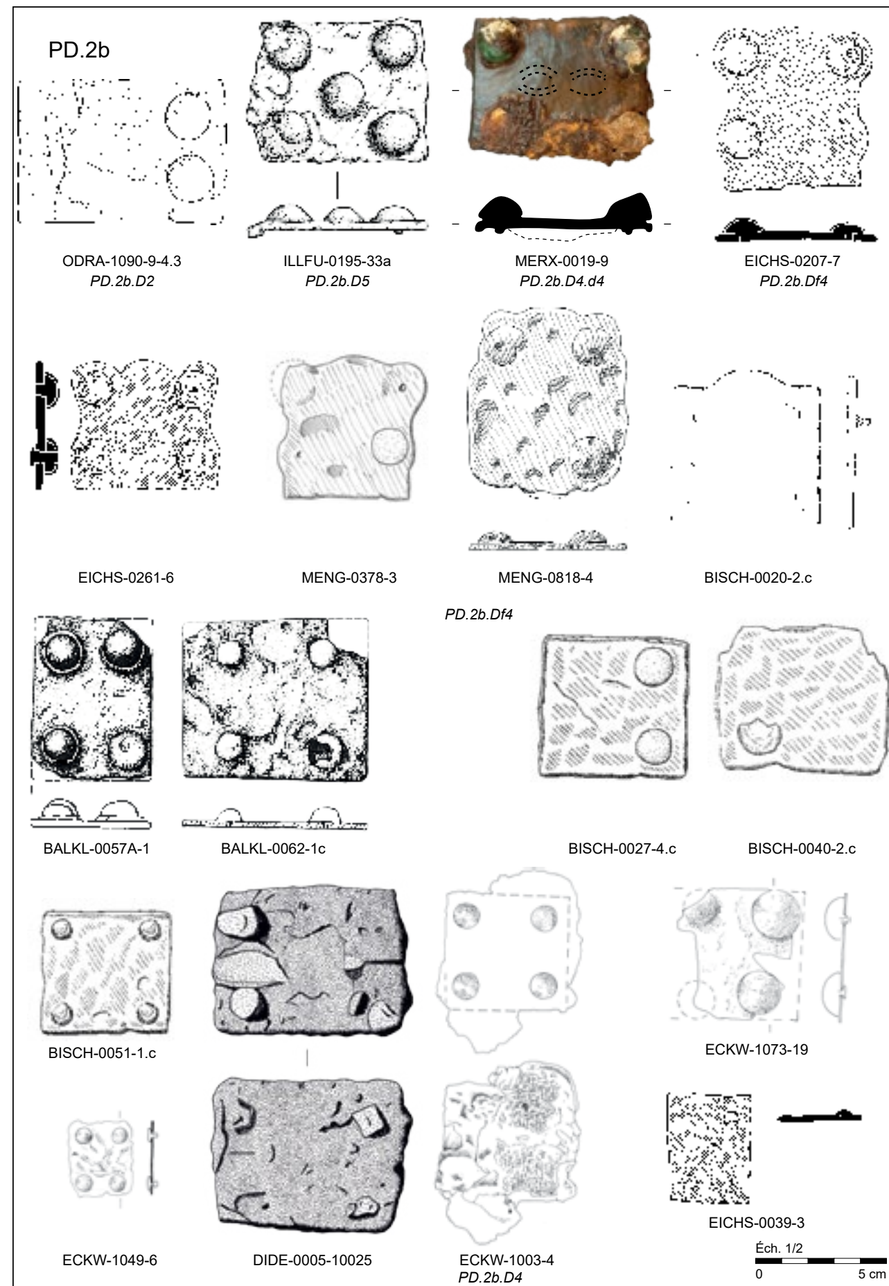
Plaques dorsales en fer non damasquiné à plaques quadrangulaires (PD.2b.D) et quadrangulaires à contours festonnés (PD.2b.Df).
