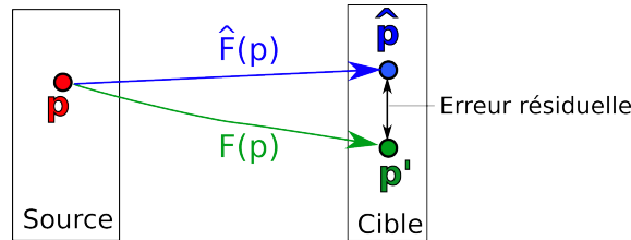
FIGURE 3.12 – Illustration de l'erreur résiduelle dans un cas d'estimation par moindres carrés ordinaires.
