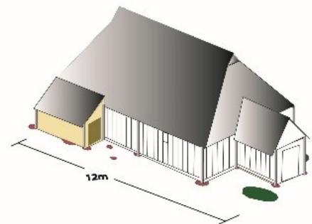
Fig. 44 : Double file de poteaux porteurs pour un plancher de grenier. Maison-étable avec stabulation au rez-de-chaussée et grange à l'étage. Crandelles, Cantal.
