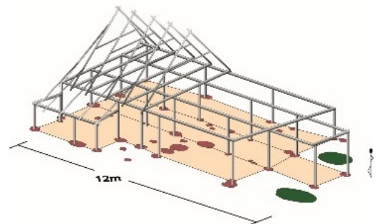
Fig. 43 : Restitution d'un bâtiment carolingien de Serris, Val d'Oise
