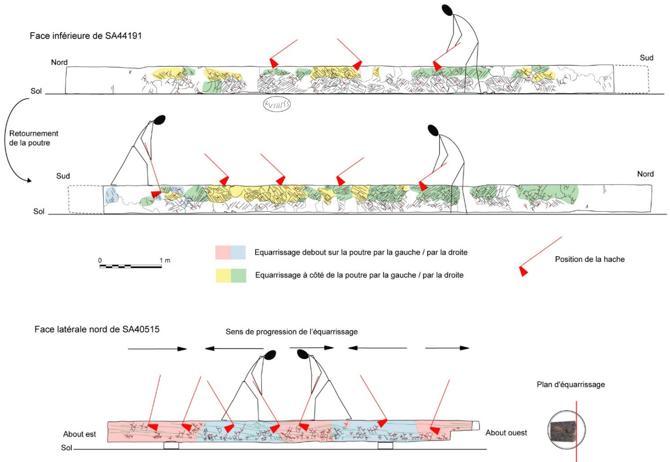
Fig. 22 : Relevé tracéologique de la face inférieure de la sablière SA44191 et de la face latérale nord de la sablière SA40515.
