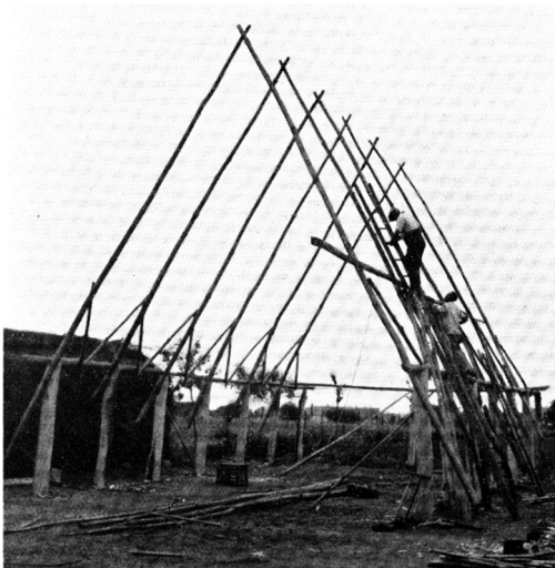
Fig. 32 : Montage d'une loge à Beaufort-en-Vallée, Maine-et-Loire (Stemmermann 1942).
