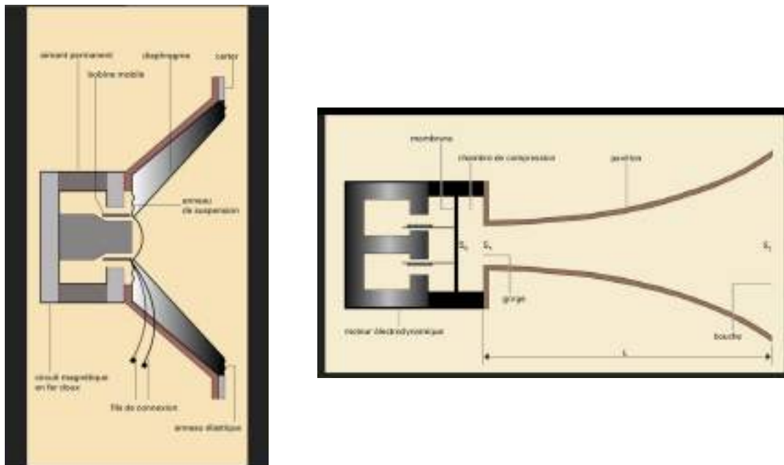
Figure 15 (à g.) un haut-parleur dit « à radiation directe » avec ses différents composants et où l'air ambiant est en contact plus important et plus directement avec la membrane. (à d.) Haut-parleur pavillon avec ses différents composants et son modèle de diffusion, la membrane est en contact limité avec l'air ambiant Illustrations extraites de Eric de Lamare ( ibid. ).
