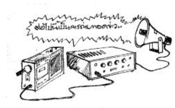
Figure 126 « Et maintenant les informations... ». A g. un poste de radio, au milieu un ampli et à droite l'enceinte. Le son filaire à Phetchabun suit ce modèle, ici simplifié. Illustration extraite de Prani (n.d. : 42).
