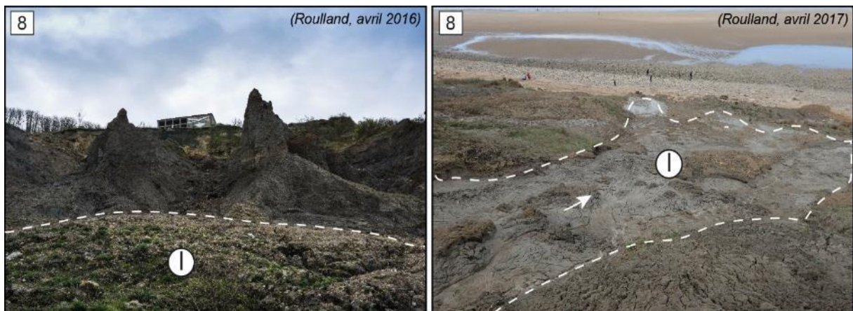
Figure 1.33 : Zone d'épandage et de coalescence des coulées de boue
