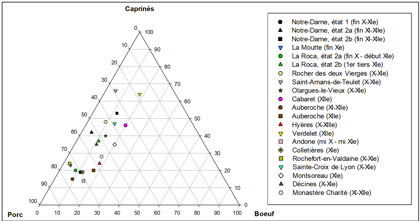
Figure 153 : Diagramme ternaire représentant les fréquences relatives des trois taxons domestiques (porcs, caprinés et boeufs) des sites élitaires de comparaison. Exprimées en %NMI.
