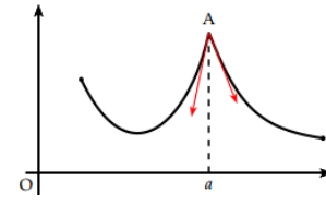
Idem. fonction non dérivable avec aussi deux demi-tangentes en A
