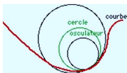
cercle osculateur à une courbe
