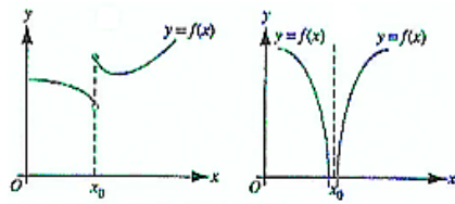
ex. de fonctions discontinues (chaque courbe n'est pas représentée en un seul morceau)
