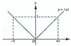
fonction non dérivable (absence d'une unique tangente au point 0)
