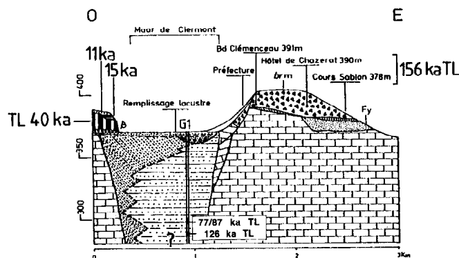
Fig. 2 - Le maar de Clermont. Croquis stratigraphique avec les différents éléments de datation. G1 : position du forage GEOCLER 1.
