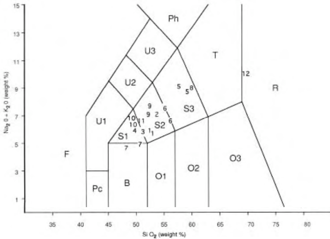
Figure 5: Chemical composition of identified tephra in SiO_2/Na_2O+K_2O (weight%) diagram (LE BAS et al. , 1985). 1 : La Moutade Tephra (2 samples). 2 : Cellule Tephra. 3 : Rouzat Upper Tephra. 4 : Rouzat Lower Tephra. 5 : Gimeaux Upper Tephra (2 samples). 6 : Les Roches Tephra. 7 : Saint-Hippolyte Tephra (2 samples). 8 : CF1 Tephra . 9 : CF2 Tephra (2 samples). 10 : CF3 Tephra (2 samples). 11 : CF4 Tephra . 12 : CF5 Tephra.
