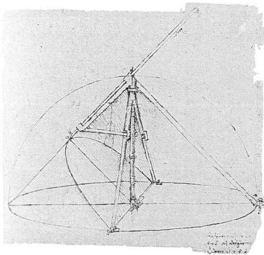
Fig. 4. Leonardo da Vinci : schéma du parabologue, 1478-1518 (Milano, Biblioteca Ambrosiana, Codex Atlanticus , fol. 394r-a).
