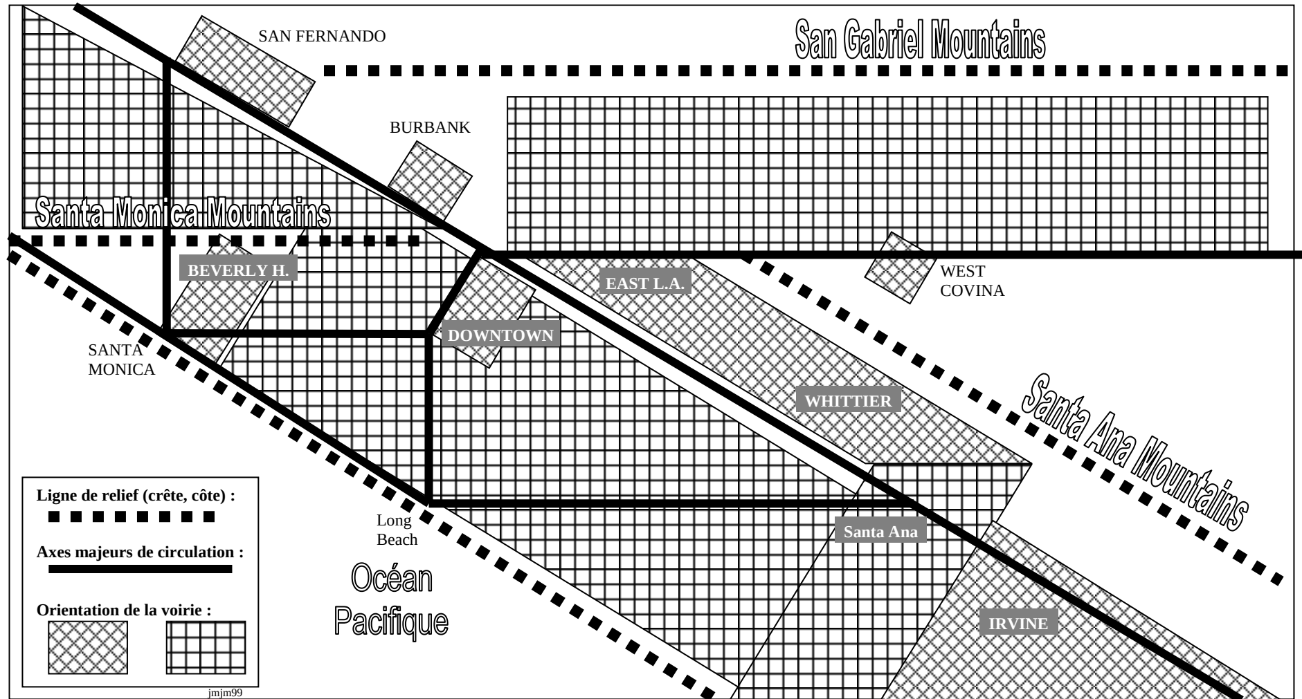
Figure 5. Schéma des structures du relief et de la voirie dans l'agglomération de Los Angeles
