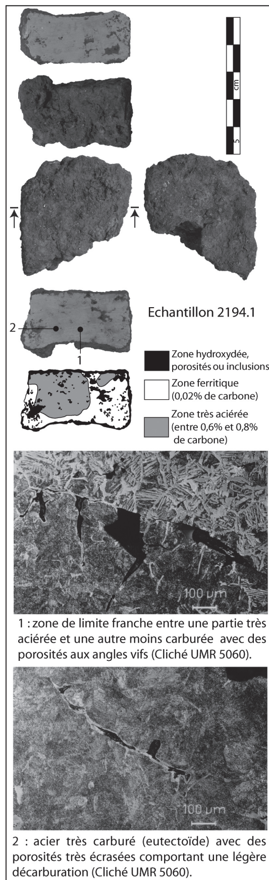
Fig. 8 : Exemple d'une étude métallographique d'un demi-produit en cours d'utilisation.
