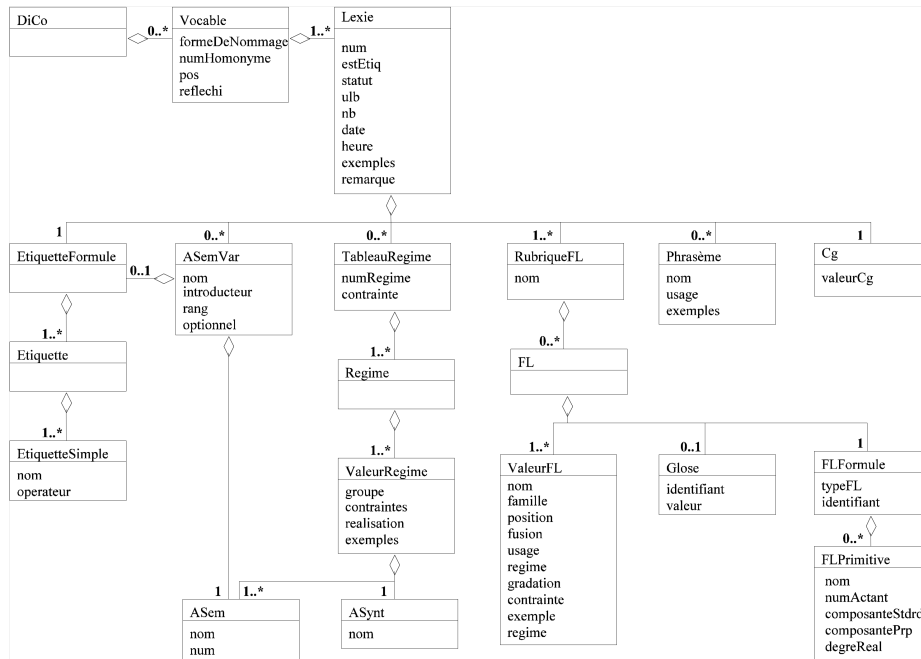
Figure 1: Modèle objet du DiCo
