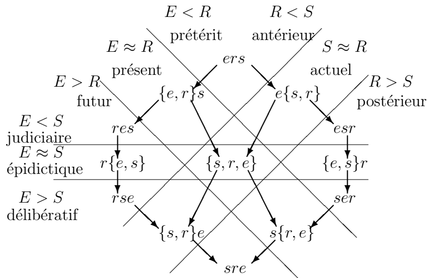
Figure 2: Le treillis Beauzée (mathématicien puis linguiste (1717–1789)) augmenté de la relation d'Aristote E/S
