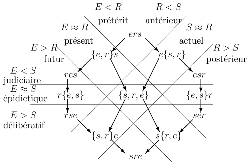
Figure 2: Le treillis Beauzée (mathématicien puis linguiste (1717–1789)) augmenté de la relation d'Aristote E/S
