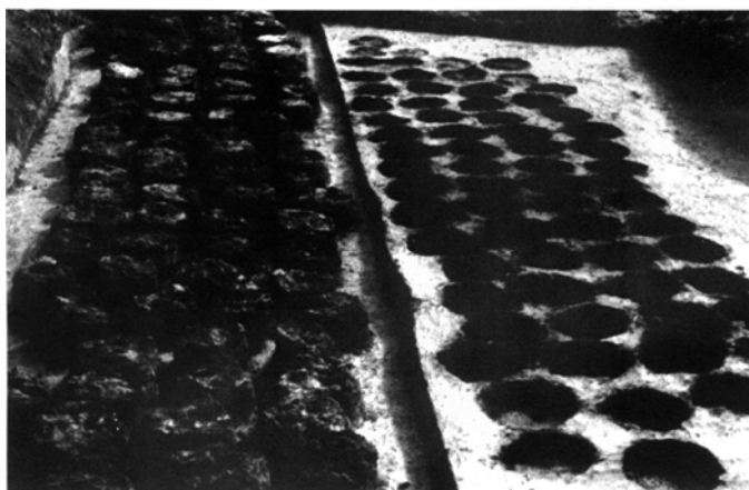
Fig. 5- Site de métallurgie du fer des Monts Sainte Croix (Pologne), caractérisé par des dizaines d'emplacements de fourneaux arasés, marqués par des fosses remplies d'un bloc de scories.
