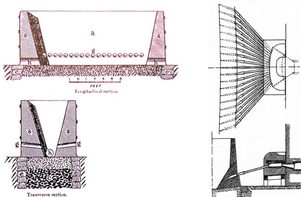
Fig. 13- Fourneau à ventilation forcée et tuyères multiples japonais « tatara »: A gauche : Coupes longitudinale et transversale du four. Source : Craddock, 1995, p. 249. A droite : Vues du système de raccord entre le soufflet et les tuyères sur un
