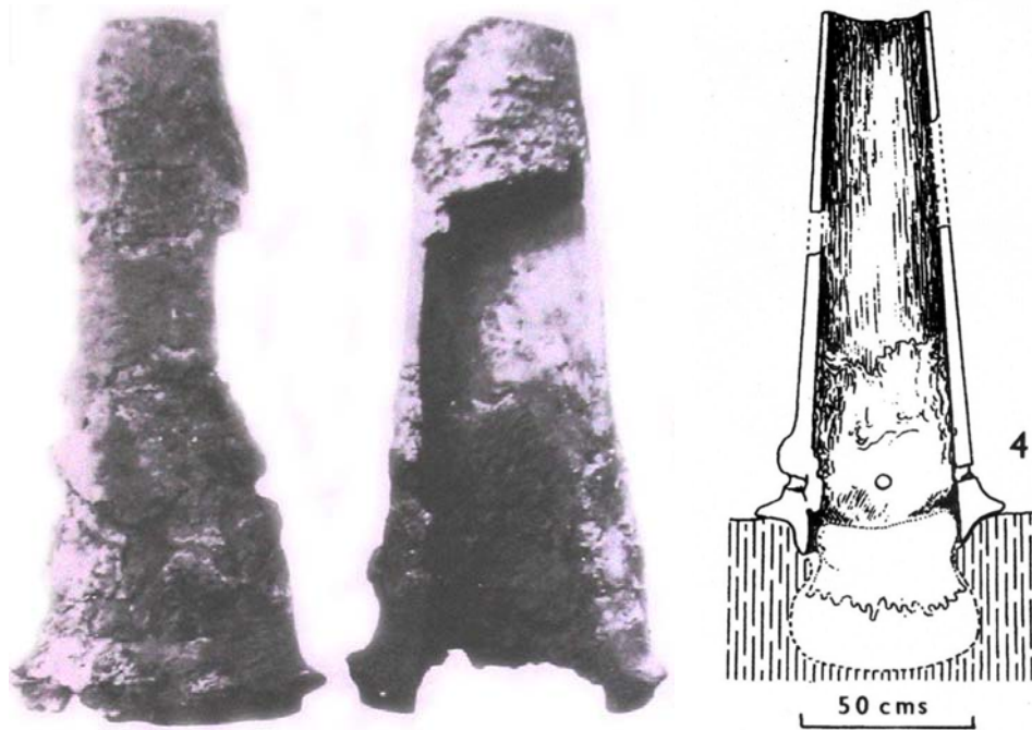
Fig. 2- Fourneau découvert à Scharmbeck (Allemagne), doté d'au moins 3 événements et régulièrement interprété comme ayant fonctionné en ventilation naturelle. A gauche : Photographies du fourneau remonté. Source : Craddock, 1995, p. 245. A droite : Restitution du four en situation. Source : Pleiner, 2000, p. 151.
