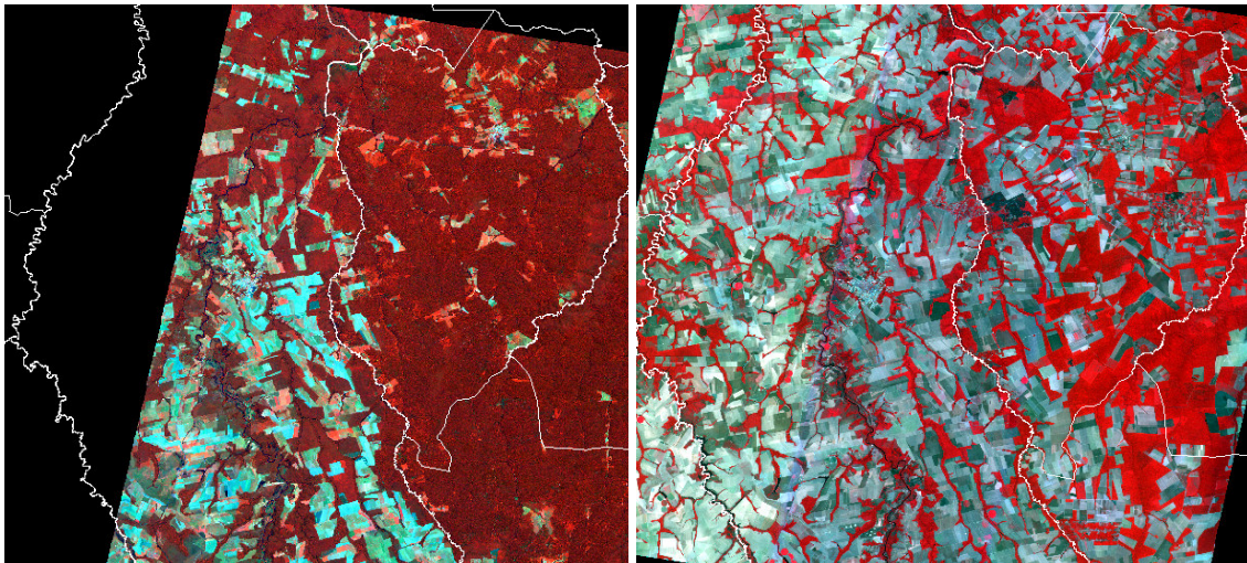
Images Landsat de 1992 (gauche) et CBERS de 2007 (droite) de la région de Sorriso-Vera
