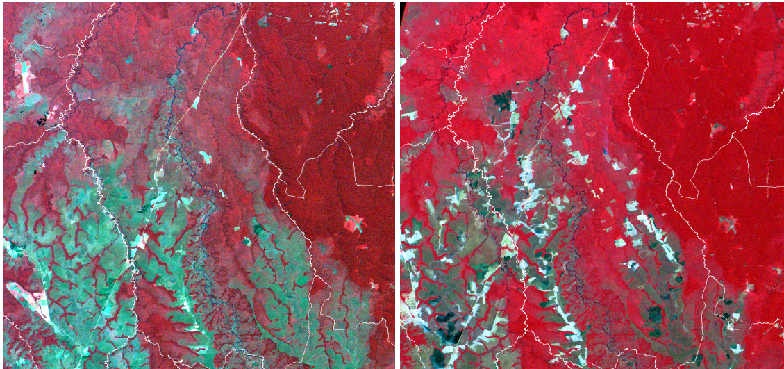
Images Landsat de 1977 (gauche) et 1981 (droite) de la région de Sorriso – Lucas do RV
