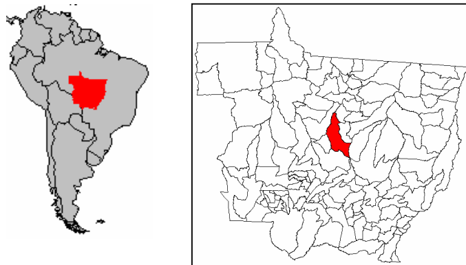
Figure 1 : Localisation du Mato Grosso et de la commune de Sorriso.(V. Dubreuil)
