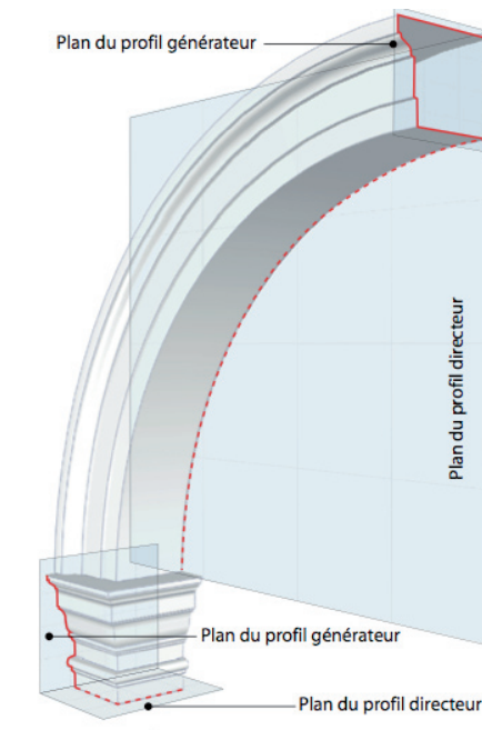
Fig. 4. Les plans de construction utilisés pour l'extraction des profils caractéristiques des formes architecturales
