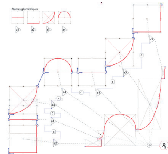
Fig. 7. Construction d'une mouleure par combinaison d'atomes géométriques
