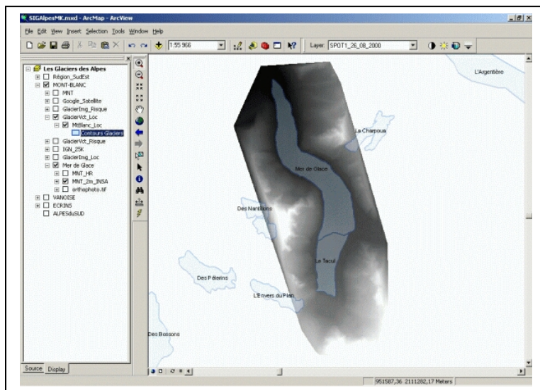
Fig.4 : Le M.N.T. haute résolution résultant Pixel de 2m. - Dégradé de niveaux de gris en fonction de l'altitude. Superposition avec localisation des glaciers.
