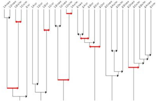
FIG. 11 Arbre cohésitif
