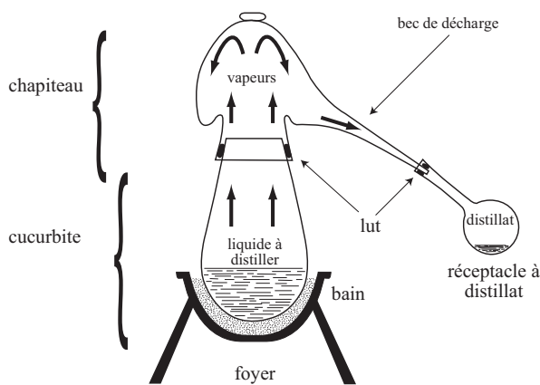
Fig. 1 : Principe de la distillation per ascensum.
