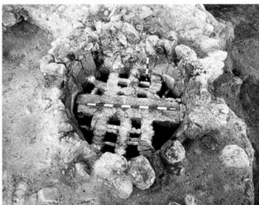
Fig. 6 Vue générale du four 250 avec sa porte fermée cuisson (Cliché M.-A. Hervás)
