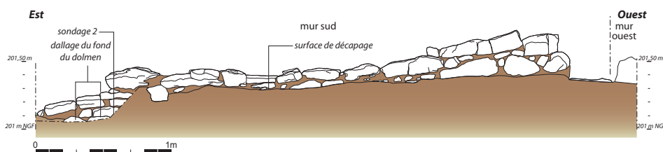
12. Mur sud élévation (DAO : F. Gueriel) / South side wall vertical section
