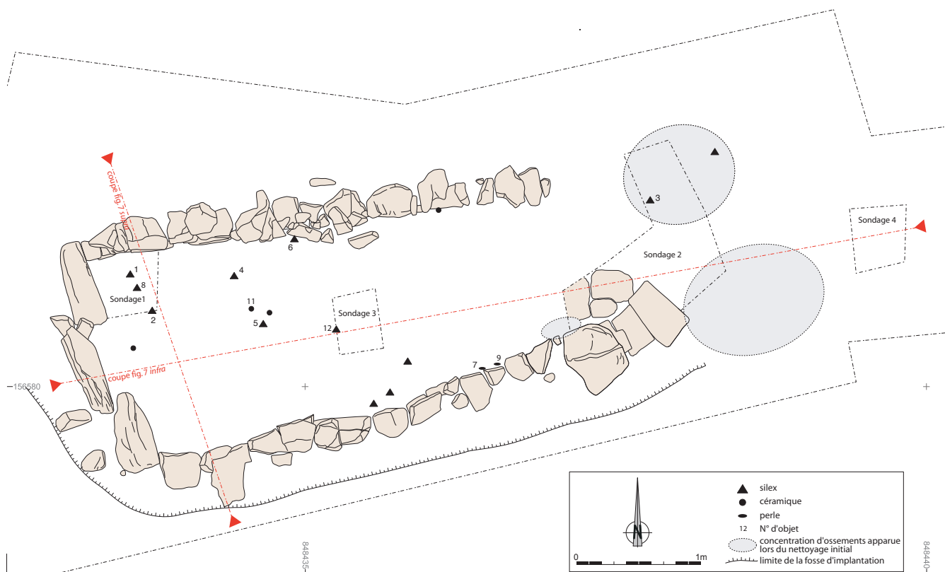
4. Plan général de la structure Pipe line Fos-Manosque-Le Puy Sainte-Réparate, Tranchée 2012, site 210 (Topo. : B. Fabry ; Relevé : P. Chapon ; DAO : P. Chapon & F. Gueriel) / The tomb ground plan
