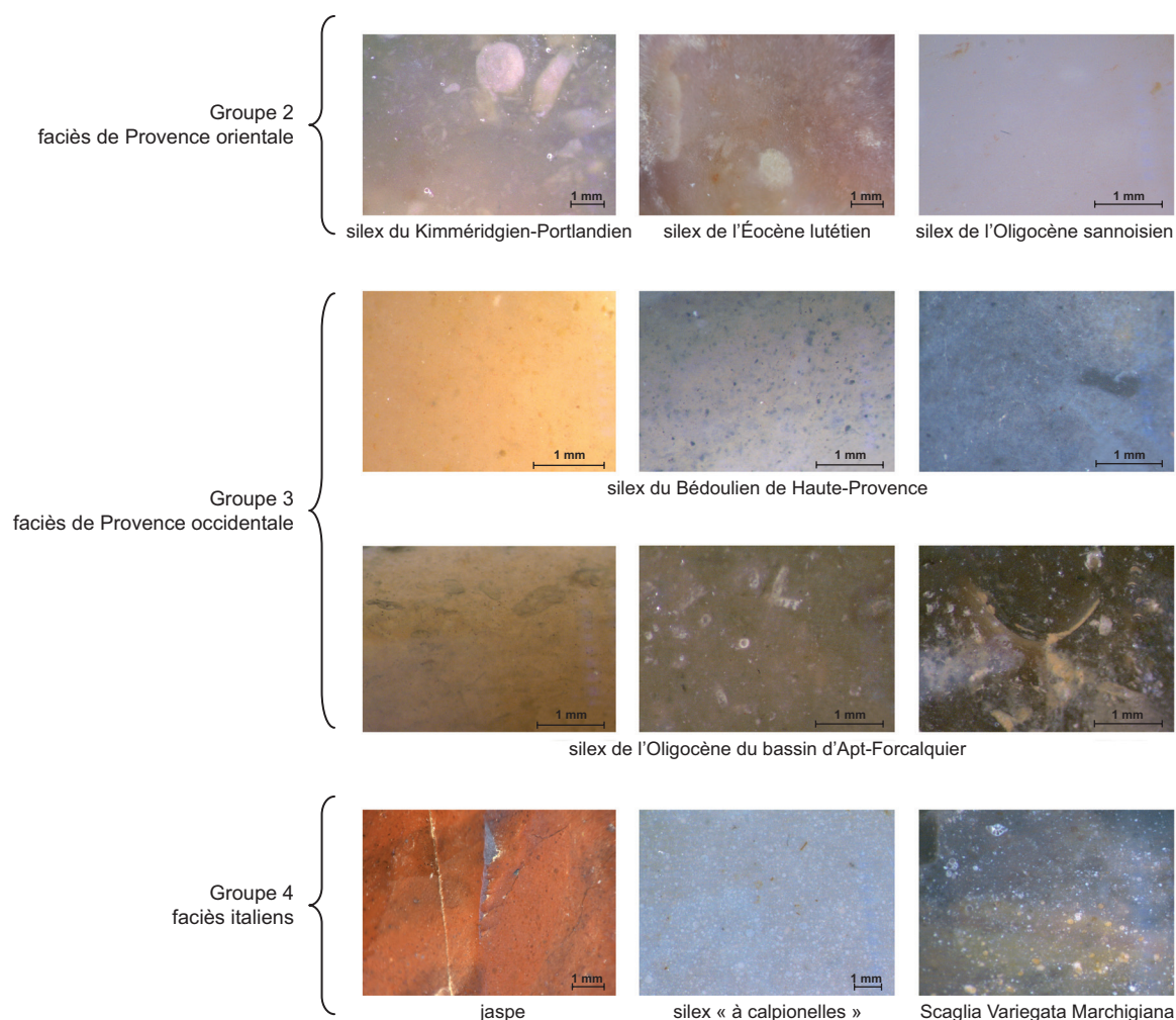
Fig. 4 – Vues macroscopiques des faciès pétrographiques individualisés à la grotte de l'Observatoire (DAO: G. Porraz, Université de Tübingen).
