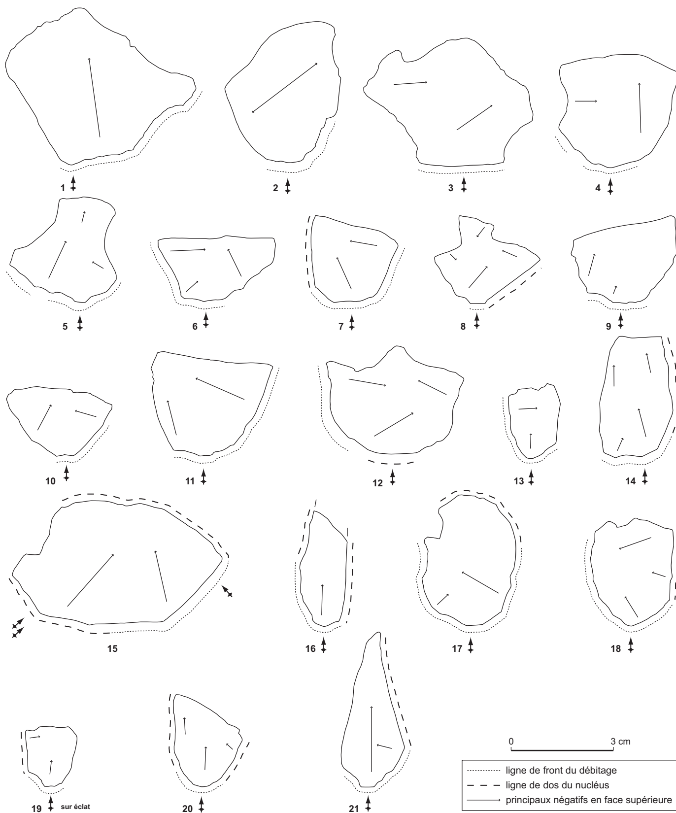
Fig. 8 – Front d'extension des débitages proto-aurignaciens « lamino-lamellaires » à la lecture des tablettes de ravivage (1, 8-14, 16, 17, 20, 21: foyer FG; 2, 3, 18: foyer F; 4-7, 19: foyer G; 15: foyers FG et G) (dessin : G. Porraz, Université de Tübingen).
