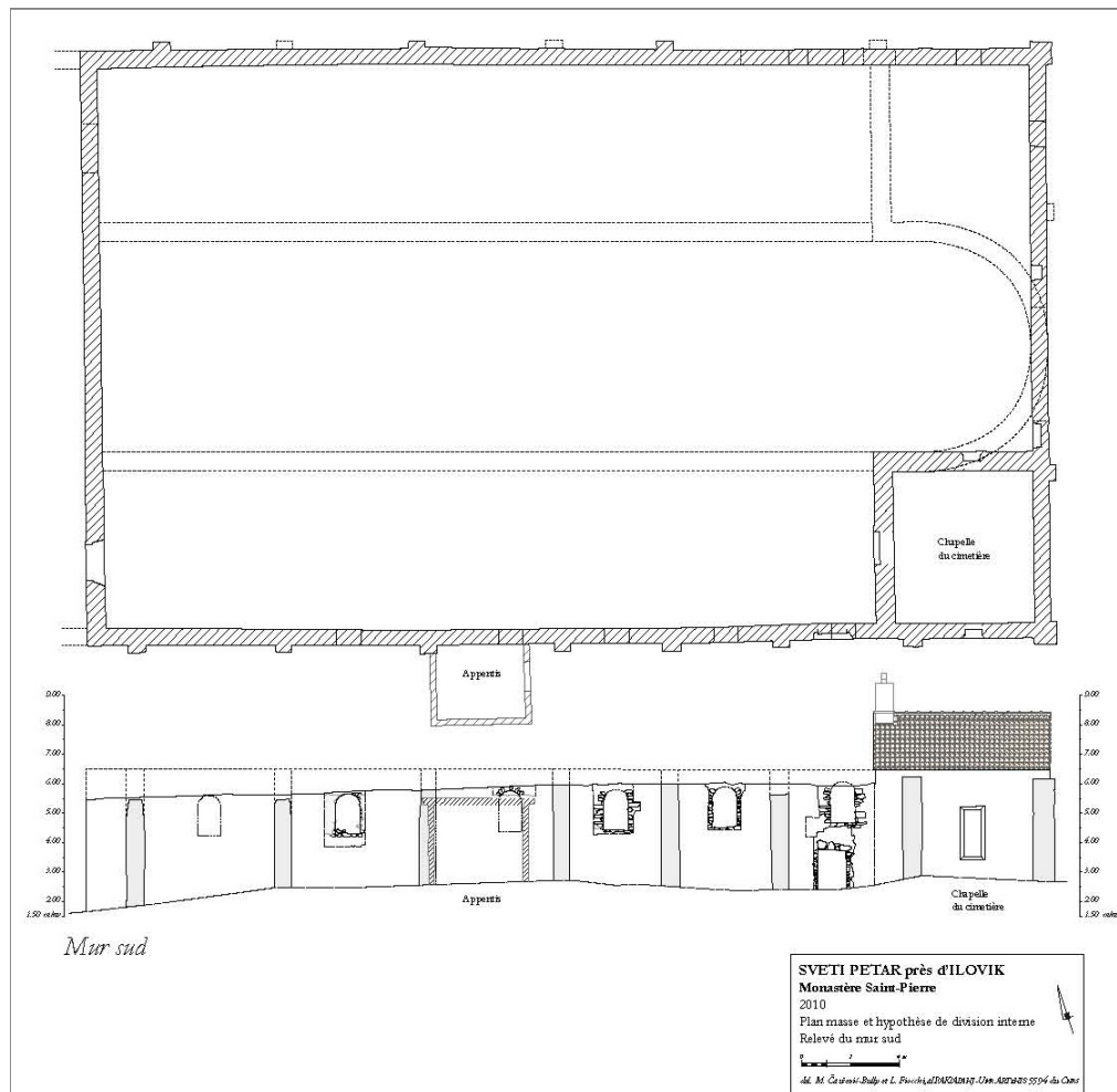
Fig. 2 - Saint-Pierre d'Ilovik, plan-masse et proposition de division interne ; relevé du mur sud (dessin M. Čaušević-Bully et L. Flocchi).
