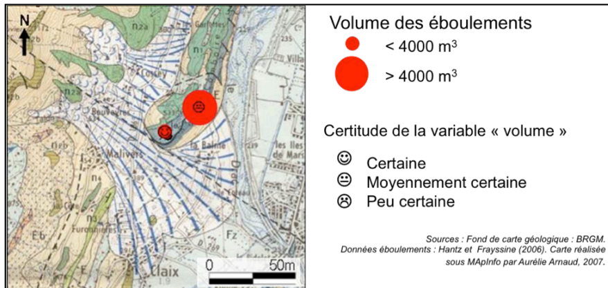
Figure 4. Cartographie des éboulements rocheux dans la couronne grenobloise : représentation de l'incertitude
