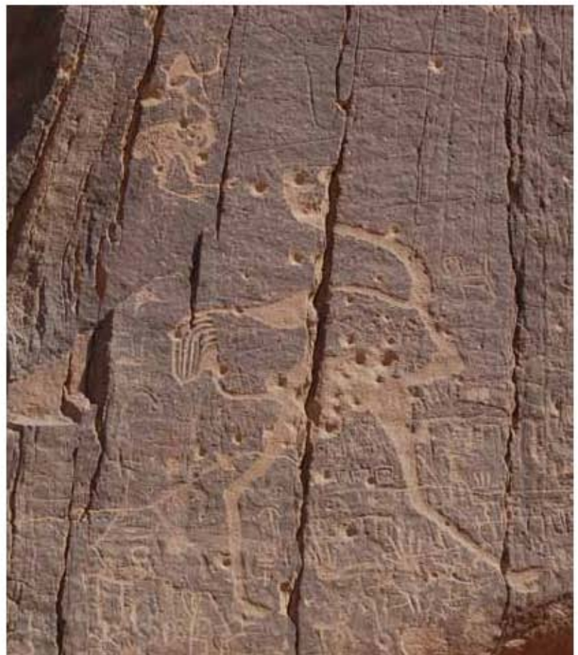
Figure 11 : panneau décoré d'une autruche à 'An an-Na'āma 2
