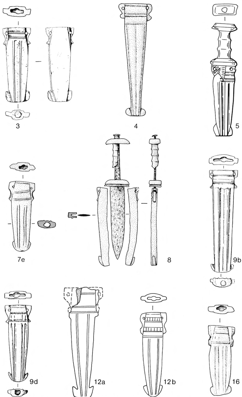
Fig. 8. Fourreaux de type 2: 3, Colchester; 4, Nydam; 5, Köln; 7e, Trier; 8, Günzburg; 9b et d, Augst; 12a et 12b, Bavay; 16, La Queue-Saint-Etienne (5, d'ap. Greep op. cit. [note 1]; 8, d'ap. W. Czysz; 9b et d, d'ap. S. Fünfschilling; 12a et b, d'ap. cat. expo. Bavay). – Éch. 2:3.
