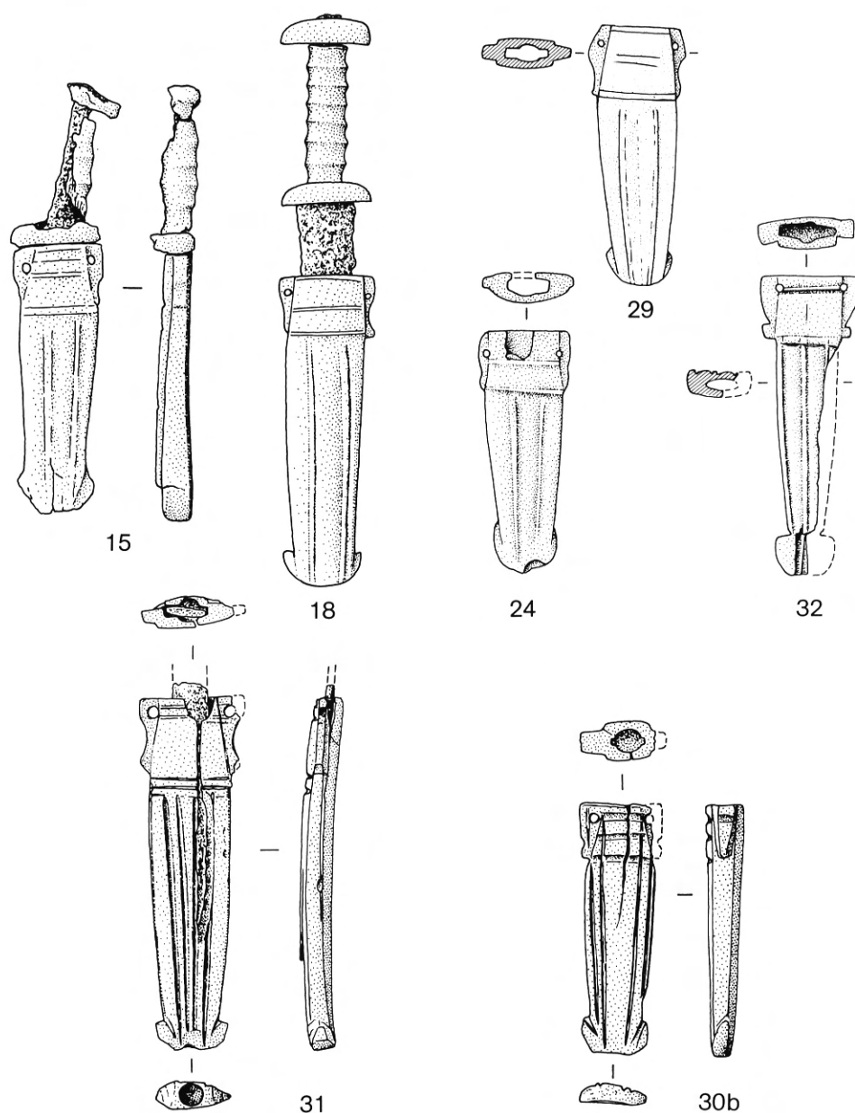
Fig.9. Fourreaux de type 2 (suite et fin): 15, Reims; 18, Saint-Marcel; 24, Clermont-Ferrand; 29, Javols; 30b, Millau; 31, L'Hospitalet; 32, Narbonne (15, d'ap. Fauduet op. cit. [note 4]; 18, d'ap. photo, ibid.; 30b et 31, d'ap. A. Vernhet). – Éch. 2:3.
