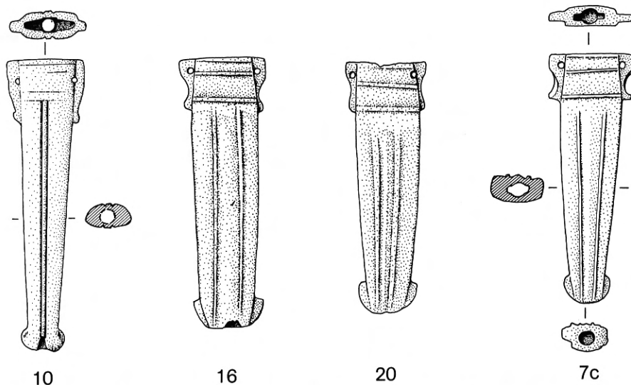
Fig. 7. Fourreaux de type intermédiaire (var. type 2): 10, Avenches; 14, Metz; 20, Alésia; 7c, Trier (10 et 20, d'ap. photos). – Éch. 2:3 (approximative pour le n° 20).
