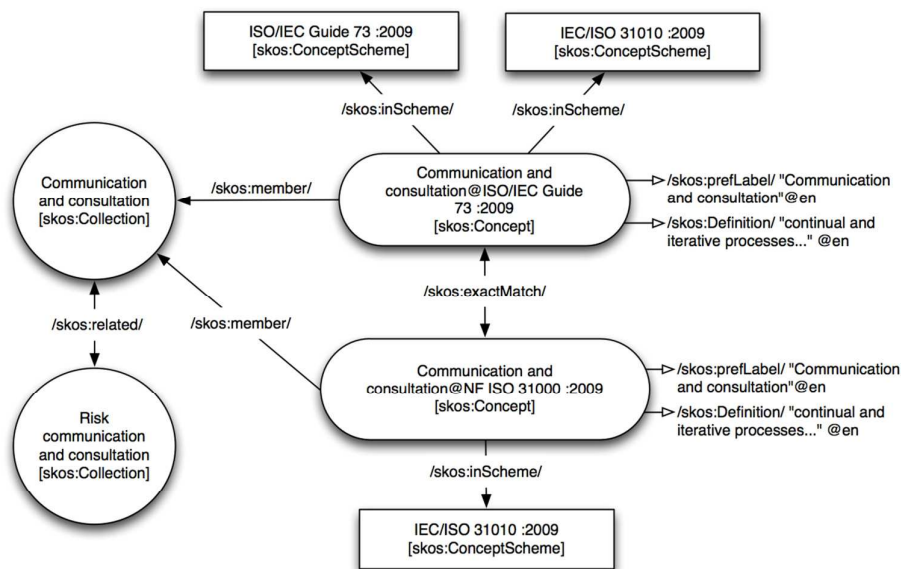
FIG. 3 – Exemple de triplets RDF dans KONTRAST.
