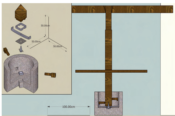
Fig. 70 – Pompéi, Pistrina . Restitution du pétrin de la maison des «Chastes amants» (IX 12, 6); éclaté isométrique et coupe (échelle 1/50; dessins N. Monteix).
