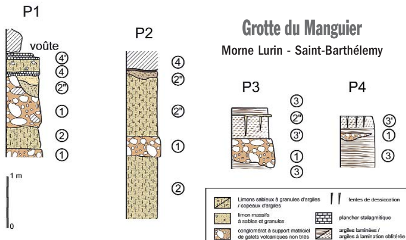
Figure 10: grotte du Manguier, lithologie des dépôts observés dans la partie profonde de la cavité.
