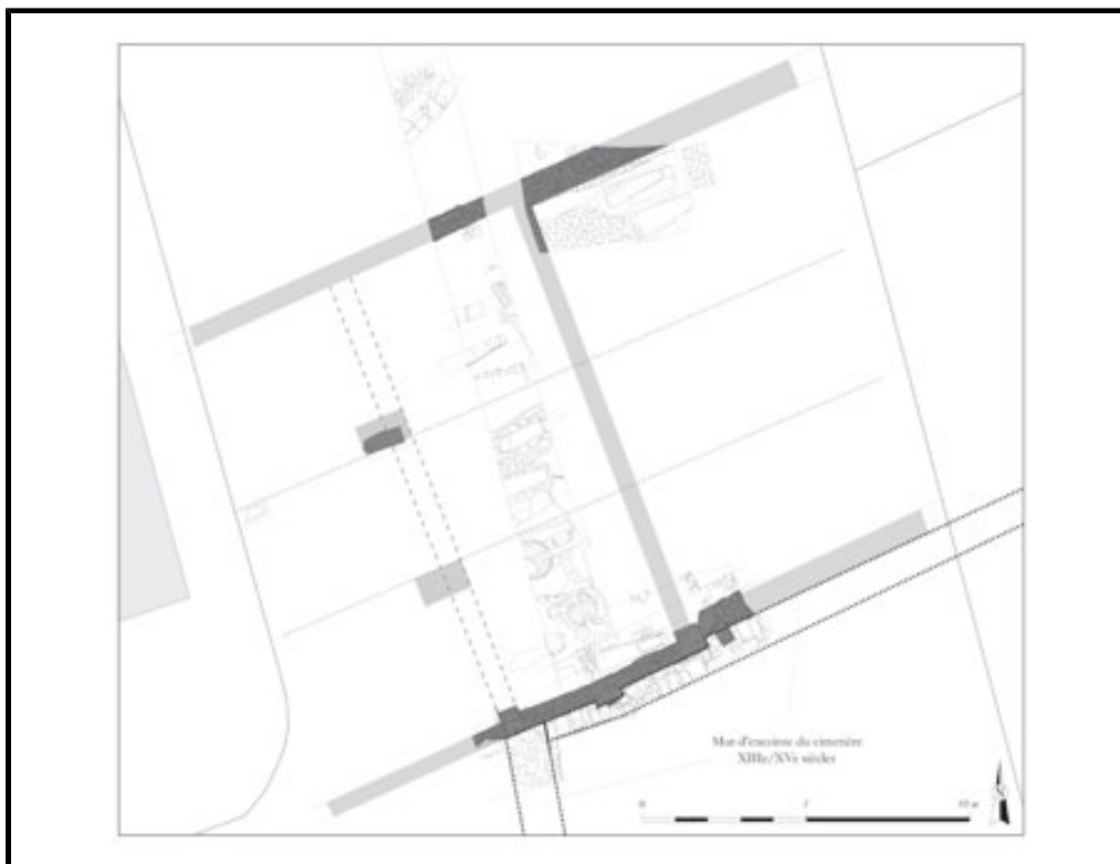
Fig. 2. Plan en partie restitué du bâtiment de la place de la Baille, d'après les données du diagnostic de 2006 (M. Dupuis).
