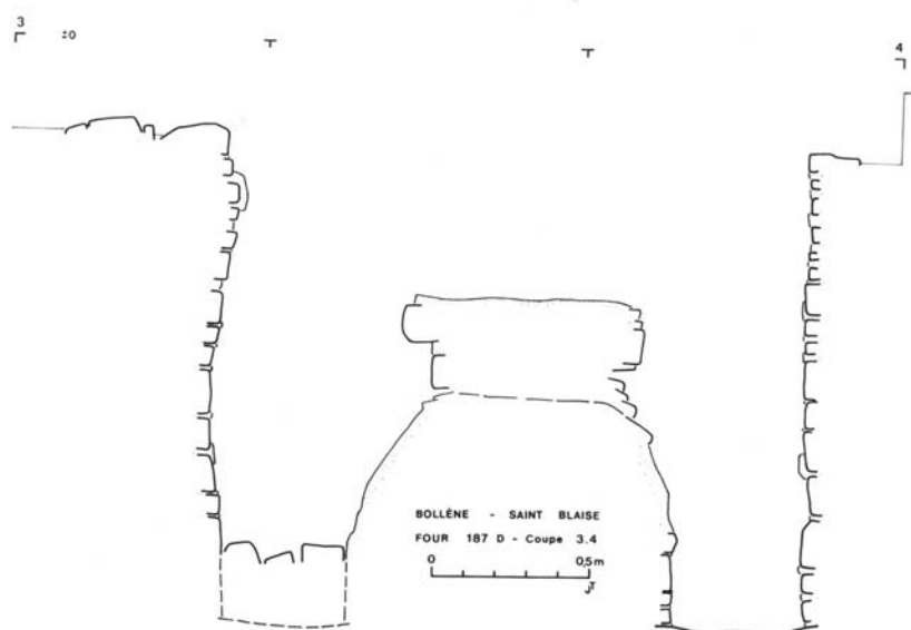
Fig. 5. — Coupe transversale 3.4.
