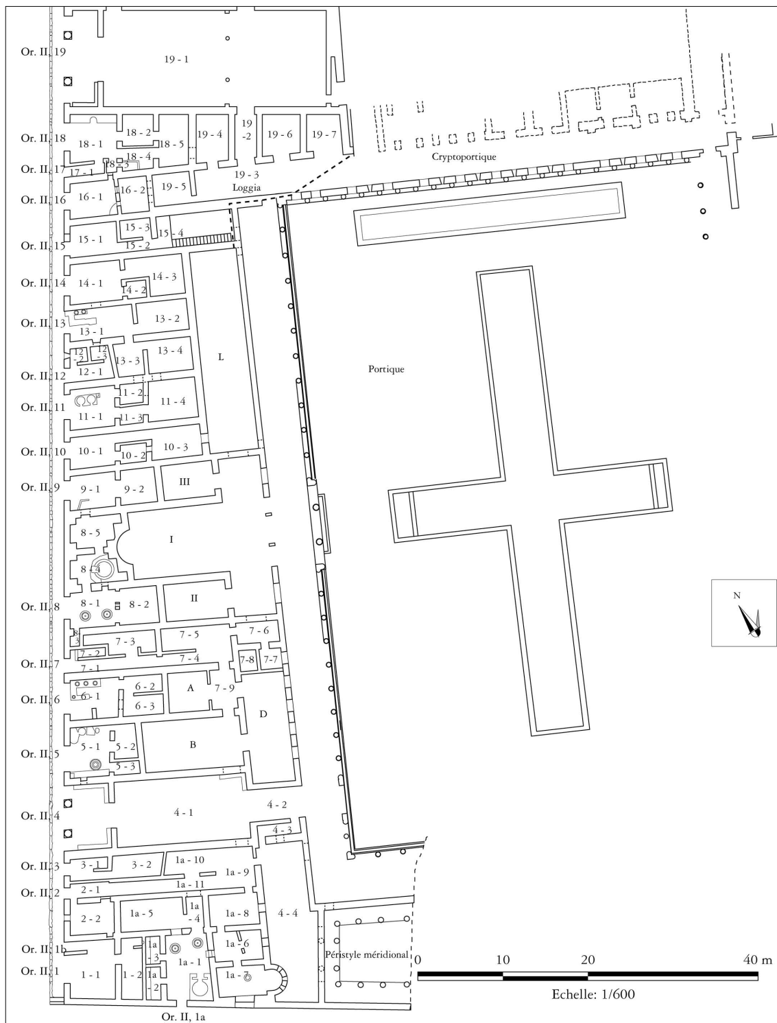
Fig. 1. Nomenclature des pièces de l' Insula Orientalis II a (DAO N. Monteix, d'après relevé F. Ferrajoli modifié par L. Trinca et M.R. Acetosio).
