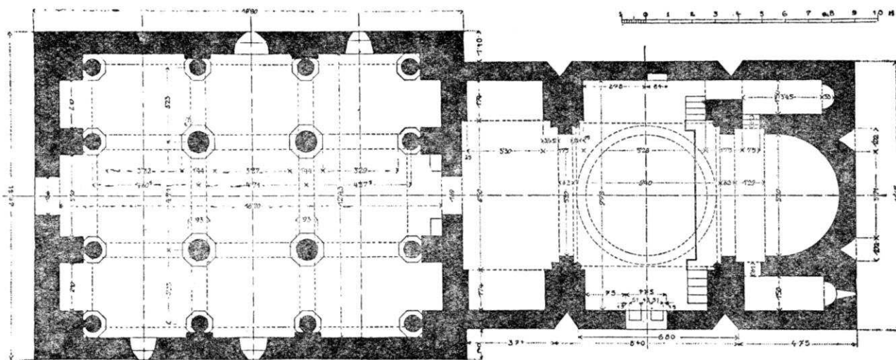
Fig. 24. Hořomos, monastère, église Saint-Jean et son gawit' ou žamatun (narthex) (d'après T'oramanyan, 1942, p. 301).
