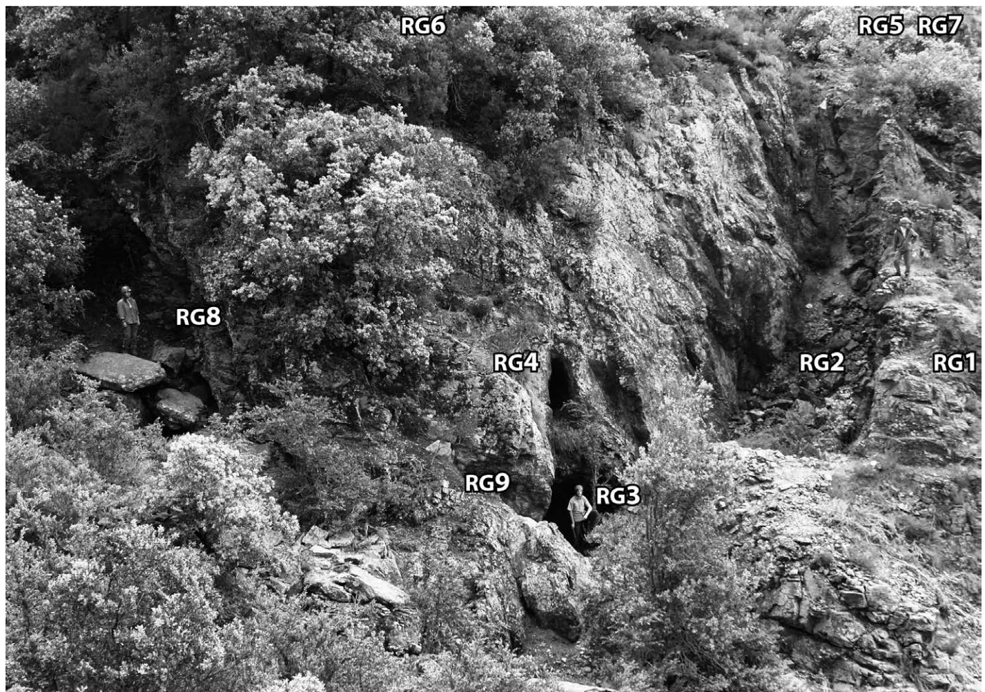
Fig. 11 Chantiers miniers en rive gauche du Colombier (cl. GEMA).
