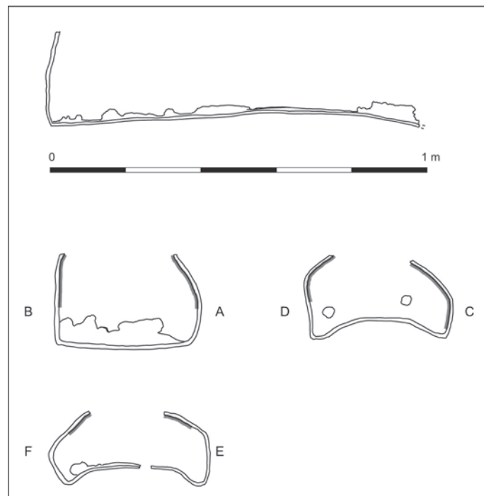
Fig. 5 – Coupe de la cuve (DAO : S. Le Maho, Inrap).
