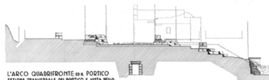
L'ARCO QUADRIFRONTI E IL PORTICO SEZIONE TRASVERSALE DEL PORTICO E VISTA DELLO STATO ATTUALE DELL'ARCO QUADRIFRONTI IN ROVI SCALA 1:50
