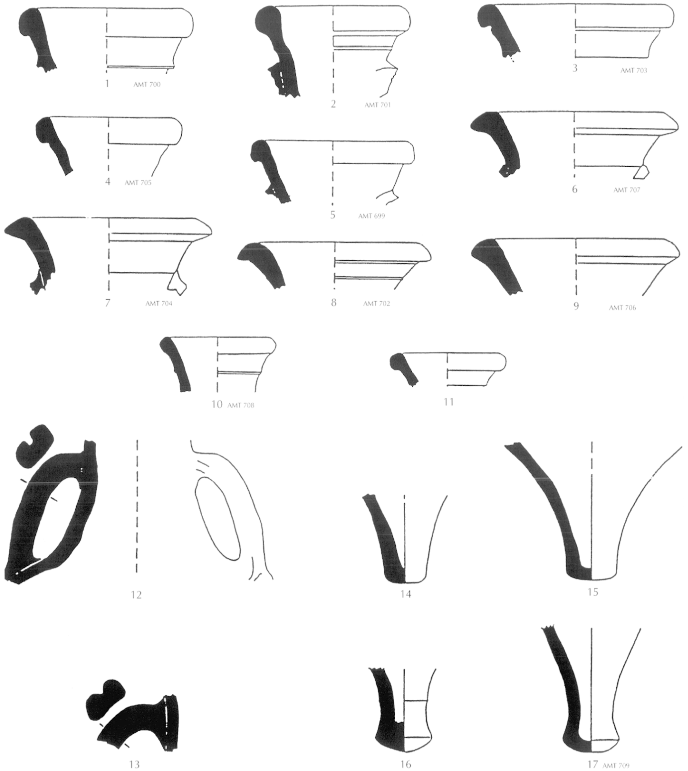
Pl. 12. Les amphores de l'atelier de la Manutention (échelle : 1/4).
