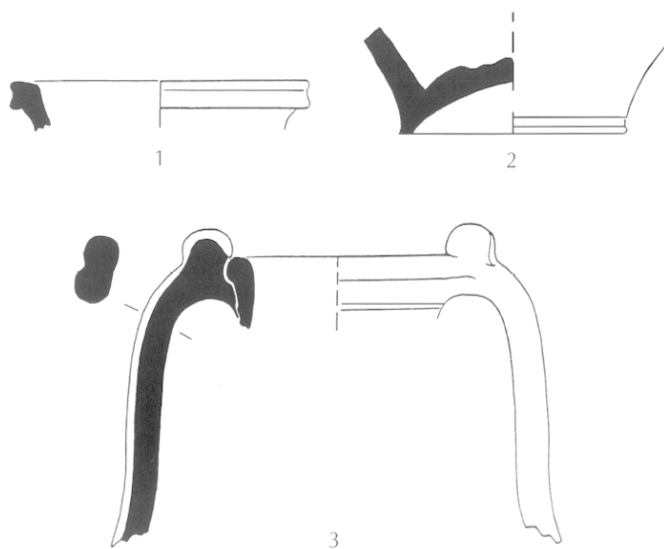
Fig. 17. Les amphores à fond plat de l'atelier de la Manutention (échelle : 1/4).
