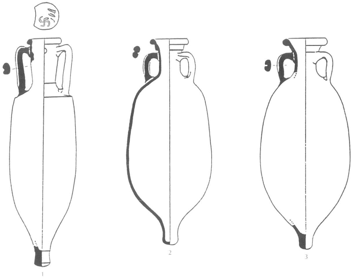
Fig. 18. Les amphores recueillies au XIX s. sur le site de la Manutention (échelle : 1/10).
