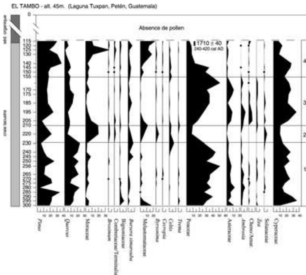
Fig. 4. El Tambo. Diagramme palynologique simplifié.
