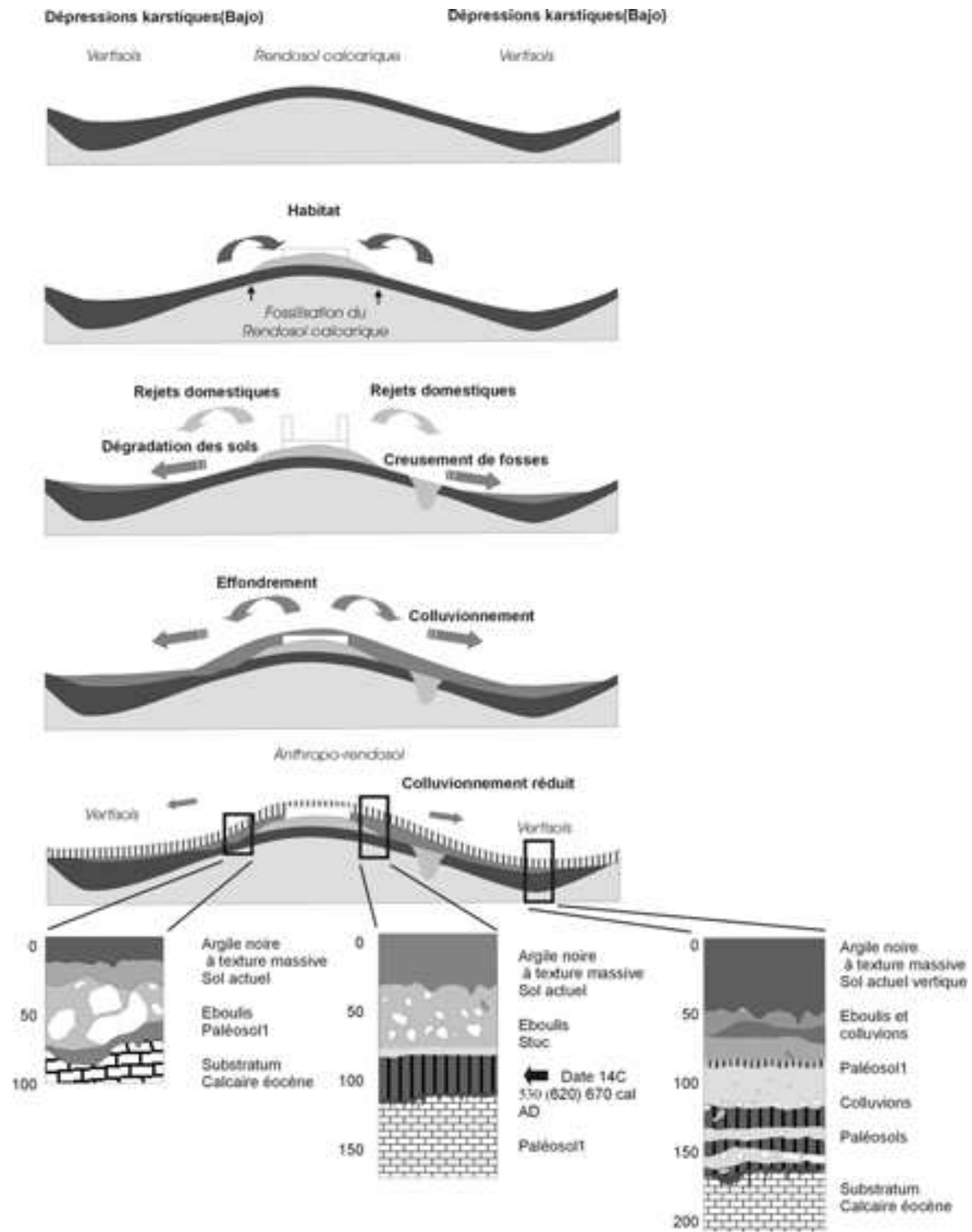
Fig. 3. Évolution pédosédimentaire synthétique du site de Gavilán.
